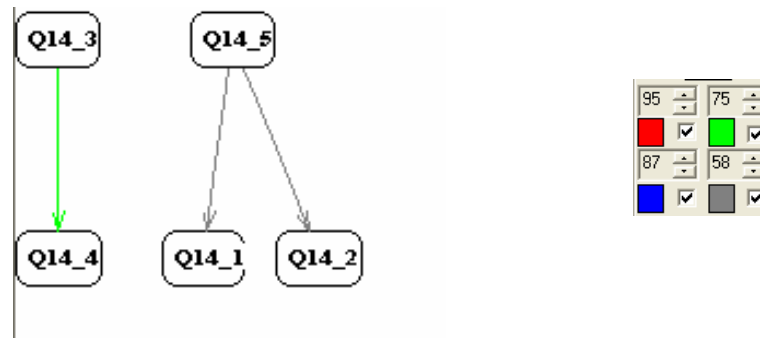
Graphique implicatif de la question 14
