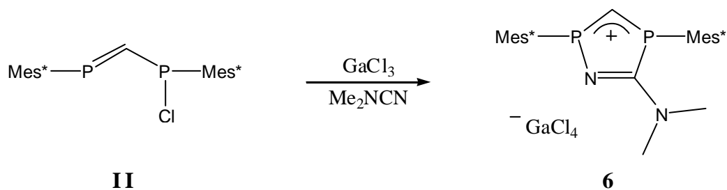
Schéma 10 : synthèse du cation 6
