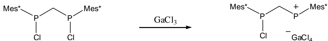
Schéma 2a : mécanisme réactionnel postulé pour la formation du cation 1
