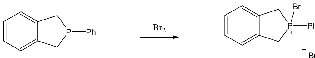
Figure 17 : oxydation d'une phosphine avec le dibrome
