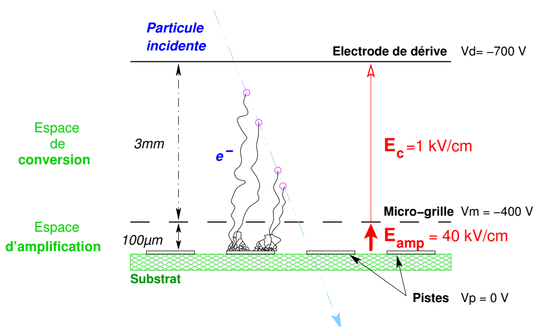
FIG. 1.1 – Principe de fonctionnement du détecteur MICROMEAS.
