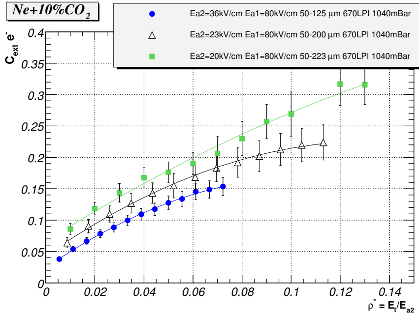
FIG. 2.16 – Coefficient d'extraction mesuré pour une grille 670 LPI pour trois gaps d'amplification (125, 200 et 220 \mu m ).
