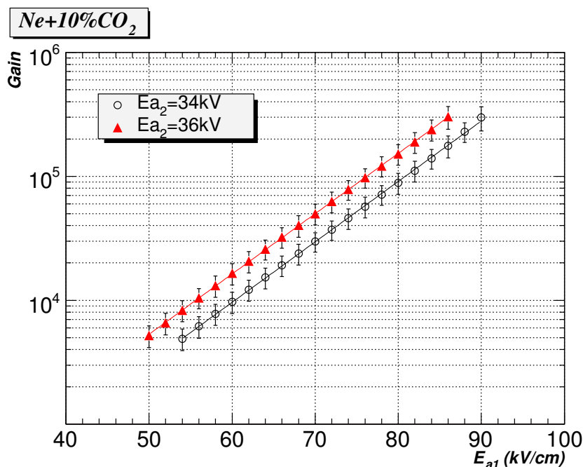
FIG. 2.19 – Gain mesuré pour la configuration 50-125 \mu\text{m} opérant avec un mélange gazeux \text{Ne}+10\%\text{CO}_2 en fonction du champ électrique E_{A1} .
