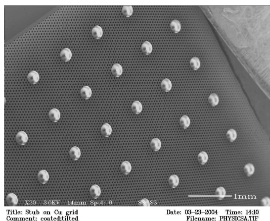
FIG. A.1 – Photographie d'une micro-grille pour MICROMEAS réalisée par l'industriel 3M.
