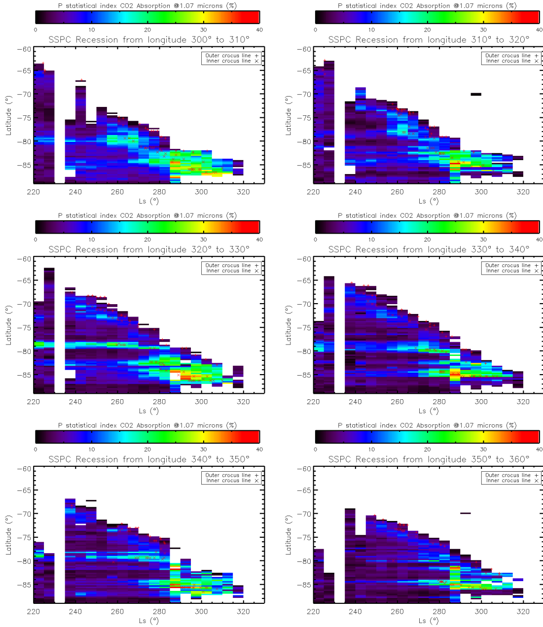
FIG. 8.21 – Évolution temporelle (en °Ls) des profils méridiens de \hat{P}_{Stat}(1 - A_{vis}) répartis entre les longitudes 300°E et 360°E. Les croix rouges représentent les lignes crocus interne et externe. Le fond de couleur correspond à la largeur de la distribution du facteur d'absorption du CO 2 à 1,07 microns mesuré par l'indicateur statistique \hat{P}_{Stat} sur les observations OMEGA.
