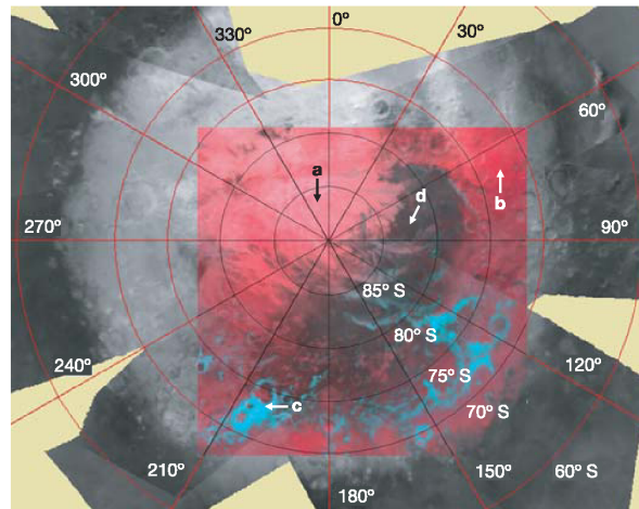
FIG. 3.4 – Classification manuelle spatiale de la calotte saisonnière sud (175). Mosaïque de 10 images OMEGA en projection stéréographique polaire sud. Les points en noir et blanc indiquent l'albédo du continuum R(1,07\mu m) . Seul l'encadré coloré ne représente pas l'albédo. La couleur rouge correspond à la profondeur de bande B_{CO_2}(1,43\mu m) . Les couleurs bleue et verte correspondent à B_{H_2O}(1,5\mu m) . La classification spatiale consiste à identifier visuellement les quatre types de terrains a, b, c et d.
