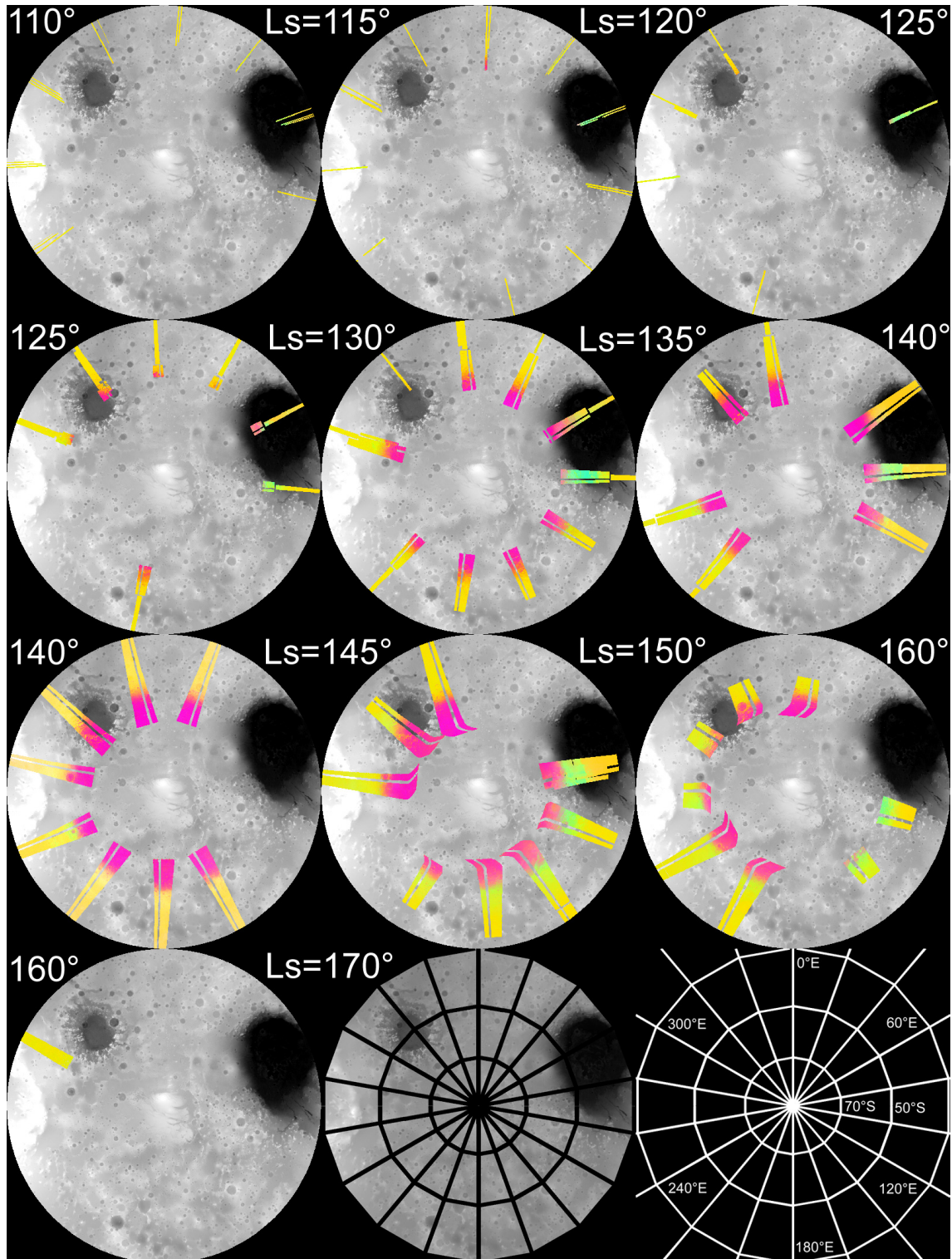
FIG. 8.1 – Carte en projection stéréographique sud de la récession de la calotte saisonnière sud entre Ls=110^\circ et Ls=170^\circ , observée par OMEGA et analysée avec la méthode Wavanglet (voir chapitre 4 page 77). Les canaux RVB correspondent respectivement aux angles de glace d'eau, de glace de CO_2 et de poussière. La couleur rouge/rose résultante correspond à la glace de CO_2 , la couleur bleue/verte correspond à la glace d'eau et la couleur jaune correspond à la poussière. Le fond en noir et blanc est la topographie MOLA, représentée seule sur l'avant dernière planche. La dernière planche représente la grille en latitude et longitude avec un pas de 20^\circ .
