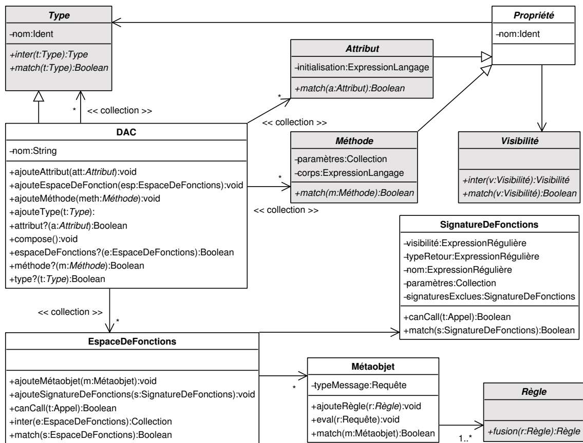
FIG. 6.5 – Résumé complet du modèle pour l'évolution structurelle et comportemental
