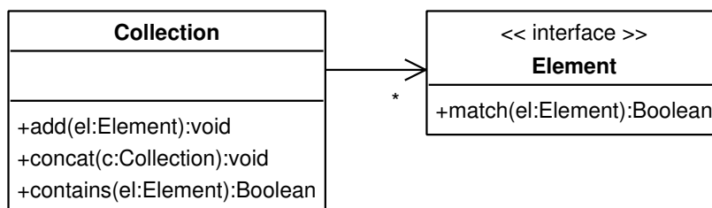
FIG. 6.2 – Le type Collection
