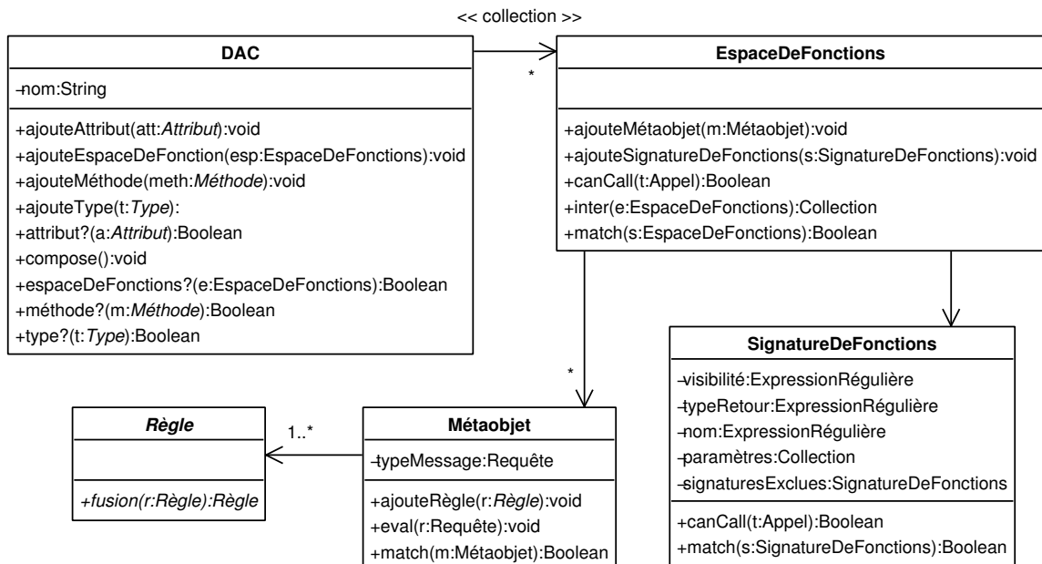
FIG. 6.4 – Métamodèle comportemental
