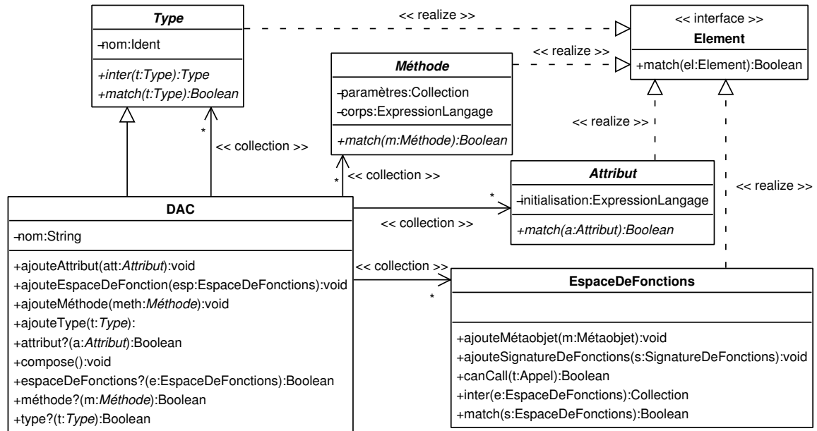
FIG. 6.1 – Description abstraite de composants
