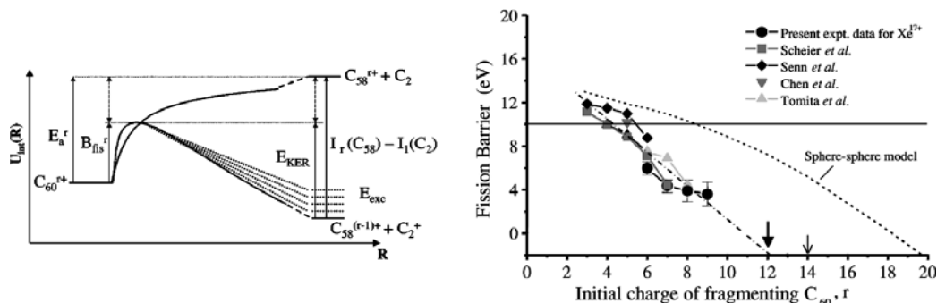
Figure 19 : Sur la gauche, schéma énergétique permettant de relier la barrière de fission asymétrique à la mesure du KER. Sur la droite, présentation des différentes mesures existantes de la barrière de fission en fonction de la charge (voir texte pour les références), ce qui permet d'extrapoler une borne inférieure de la limite de stabilité du C_{60} par un calcul semi-empirique ; la borne supérieure étant donnée par un « over-the-barrier model ». Les flèches dénotent la prédiction théorique (flèche normale) et la valeur expérimentale (flèche grasse) de référence actuellement.
