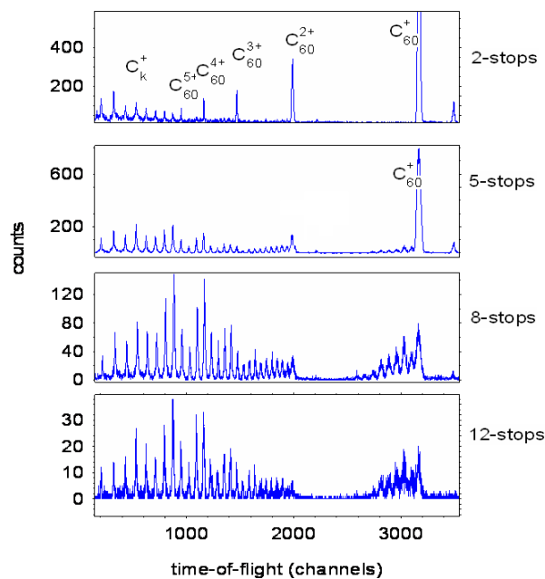
Figure 33 : Spectres « n stops » ( n = 2, 5, 8 et 12 ) obtenus après analyse du spectre de temps de vol lié aux collisions (C_{60})_n + Xe^{30+} @ 600 keV ( T_{four} = 525 °C).
