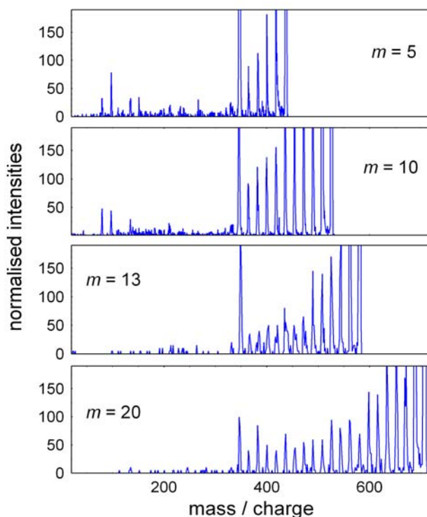
Figure 55 : Spectres de fragmentation des anions d[AMP(H_2O)_m]^- pour différents nombres m de molécules d'eau attachées, suite à des collisions de 50 keV sur des atomes de sodium neutres. Les intensités ont été normalisées en fonction du comptage total.
