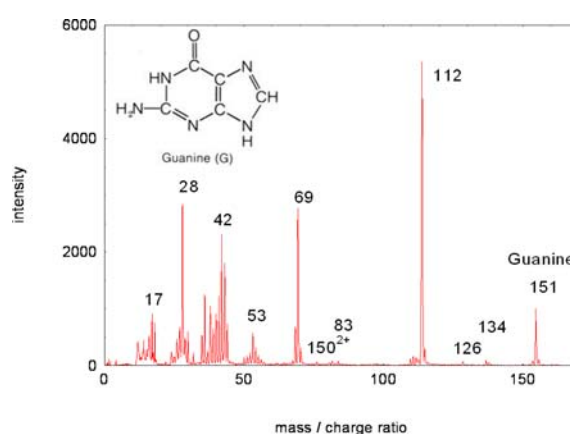
Figure 43 (données non publiées): Spectre de fragmentation de la guanine en phase gazeuse suite à des collisions avec des ions O^{5+} @ 50 keV. A notre connaissance, aucune autre étude en phase gaz de cette molécule a été réalisée à ce jour.
