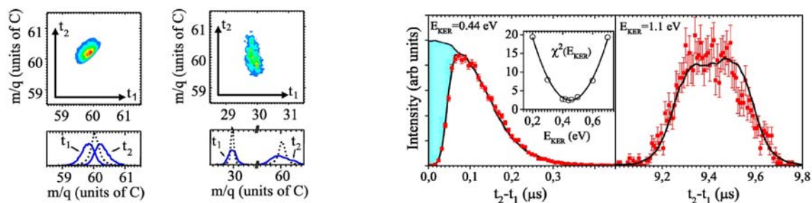
Figure 36 : Sur la gauche, deux parties du spectre de corrélation à « 2 stops » liées aux processus de fission (C_{60})_2^{2+} \rightarrow C_{60}^{+} + C_{60}^{+} et (C_{60})_2^{3+} \rightarrow C_{60}^{2+} + C_{60}^{+} . Les distributions simulées en temps de vol des deux fragments, respectivement t_1 et t_2 , sont représentées en dessous ; à titre de comparaison, les distributions en pointillées, qui sont celles liées aux événements de simple capture électronique de monomères présents dans le spectre à « 1 stop », sont indiquées. Sur la droite, les spectres de différence en temps de ces deux fissions sont donnés. Les données expérimentales (en rouge) et simulées (trait noir) sont comparées, permettant d'extraire de la simulation le KER lié au processus de fission. Dans le processus (C_{60})_2^{2+} \rightarrow C_{60}^{+} + C_{60}^{+} , la zone en bleu représente les événements non détectés expérimentalement, à cause du temps mort de détection et l'insère montre l'optimisation du KER par ajustement statistique (voir texte).
