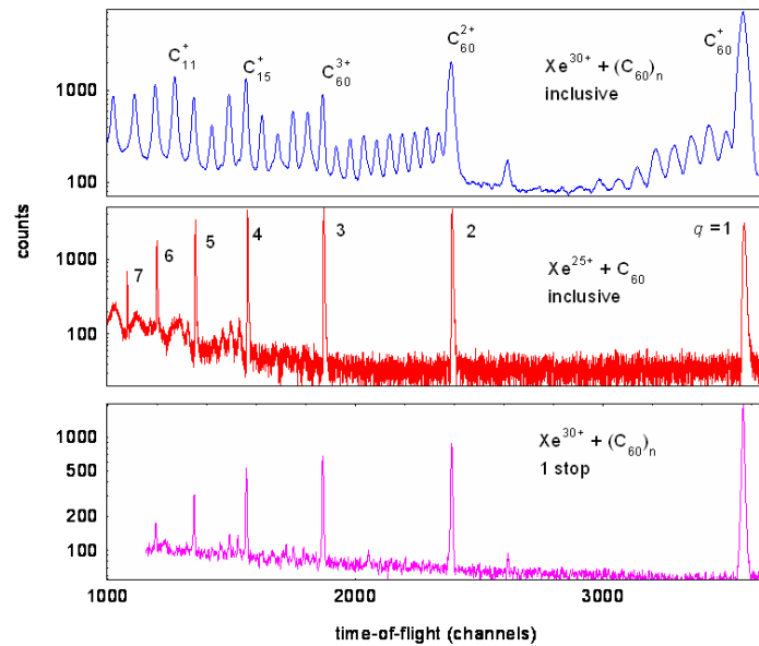
Figure 32 : En haut, première partie du spectre inclusif (ensemble des multiplicités) de temps de vol obtenu suite à des collisions (C_{60})_n + Xe^{30+} @ 600 keV ( T_{four} = 590 °C). Au centre, spectre inclusif de temps de vol obtenu dans des collisions C_{60} + Xe^{25+} @ 500 keV. En bas, première partie du spectre « 1 stop » (contenant seulement les événements de multiplicité 1) issu de l'analyse du premier spectre (en haut).
