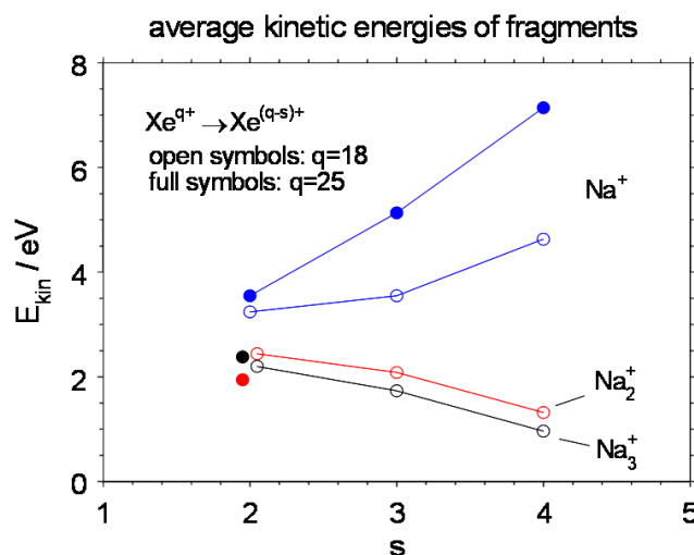
Figure 14 (données non publiées) : Mesures de l'énergie cinétique, en fonction du nombre d'électrons stabilisés sur le projectile, des fragments légers et monochargés émis lors de la multi-ionisation d'agrégats de sodium par des ions de xénon chargés 18 et 25 fois, de basse énergie.
