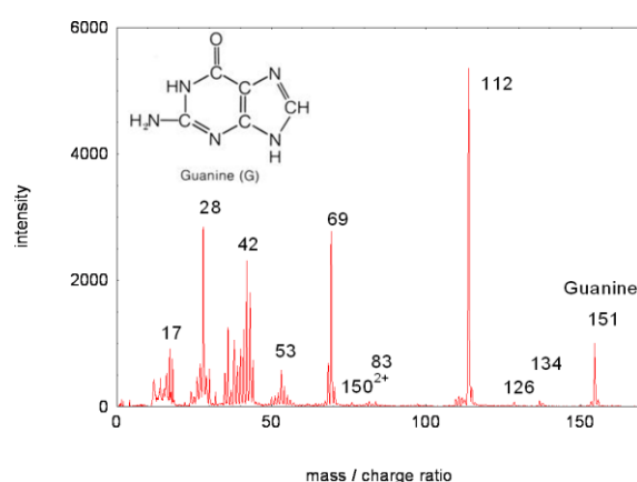
Figure 43 (données non publiées): Spectre de fragmentation de la guanine en phase gazeuse suite à des collisions avec des ions O^{5+} @ 50 keV. A notre connaissance, aucune autre étude en phase gaz de cette molécule a été réalisée à ce jour.
