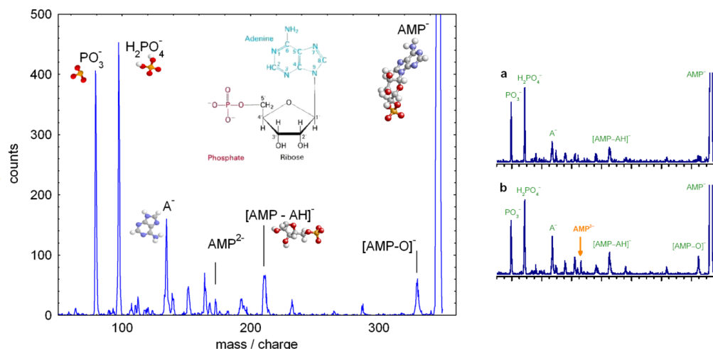
Figure 54 : A gauche, spectre de fragmentation obtenu suite à des collision d'AMP à 50 keV sur des atomes de sodium neutres ; les voies principales de dissociation sont indiquées. A droite, comparaison des spectres de fragmentation suite à des collisions sur des atomes de néon (en haut) et de sodium (en bas). Dans le premiers cas, seules les voies de dissociation par CID sont ouvertes.
