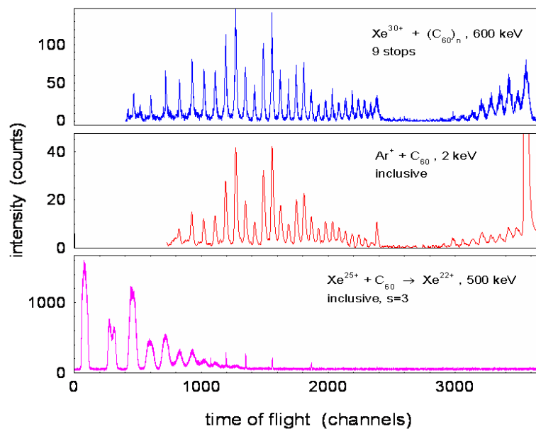
Figure 35 : En haut, spectre « 9 stops » obtenu suite à des collisions (\text{C}_{60})_n + \text{Xe}^{30+} @ 600 keV ( T_{\text{fuser}} = 590 °C). Au centre, spectre de masse observé suite à des collisions \text{C}_{60} + \text{Ar}^+ @ 2 keV. En bas, spectre de masse observé suite à des collisions \text{C}_{60} + \text{Xe}^{25+} @ 500 keV, où trois électrons ont été stabilisés sur le projectile, ce qui correspond à une multi-ionisation du \text{C}_{60} ; le laissant dans un état de charge moyen de 9.
