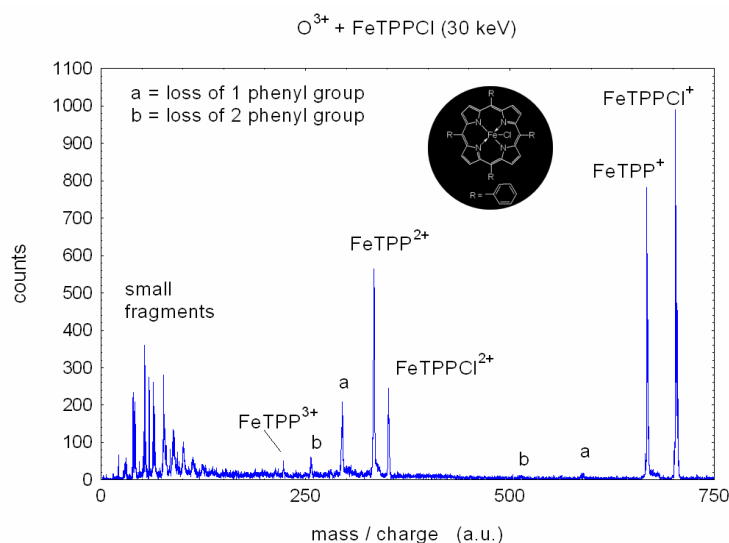
Figure 45 (données non publiées) : Spectre de fragmentation de la FeTPPCI suite à des collisions avec des ions \text{O}^{3+} @ 30keV. Les voies de dissociation majoritaire montre la perte soit de l'atome de chlore, soit d'un ou plusieurs groupes phényle.
