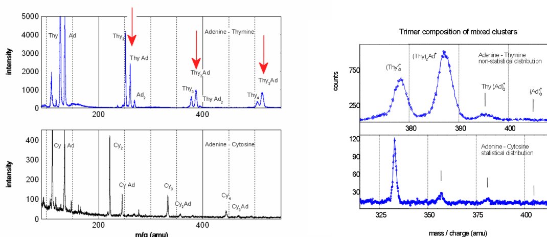
Figure 65 (données non publiées) : A gauche, partie des spectres de masse d'agrégats mixtes chargés de (Ad/Thy) et (Ad/Cy) , obtenus dans des collisions avec des ions O^{5+} @ 50 keV. Dans le premier cas (en haut), l'agrégation ne semble étonnamment pas statistique comme le montre la prédominance des pics signalés par les flèches rouges (voir texte). A droite : zoom sur la composition du groupe trimère dans les cas précédents, insistant sur la différence dans le processus d'agrégation.
