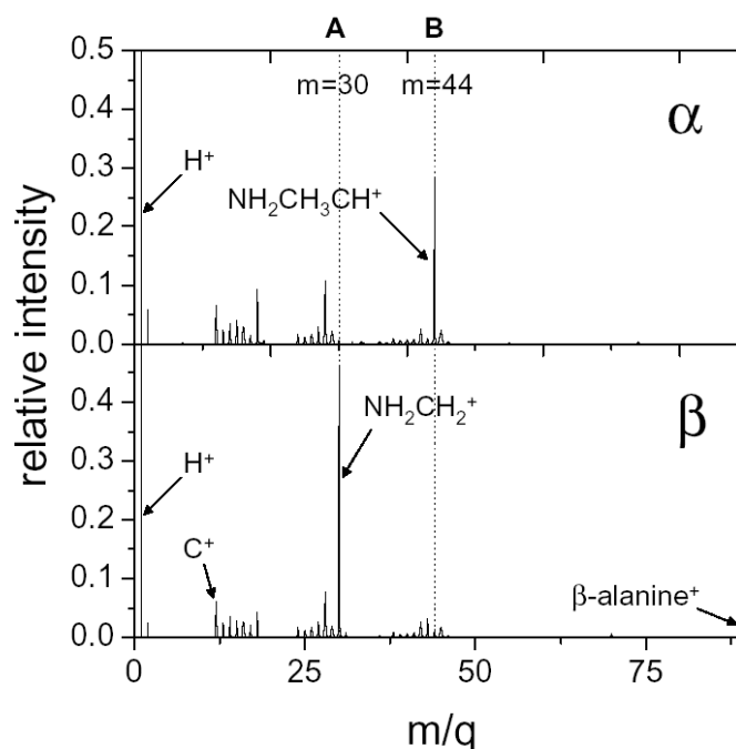
Figure 48 (données non publiées) : Spectres de fragmentation de \alpha -Ala (en haut) et \beta -Ala (en bas), suite à des collisions avec des ions He^{2+} @ 40 keV.
