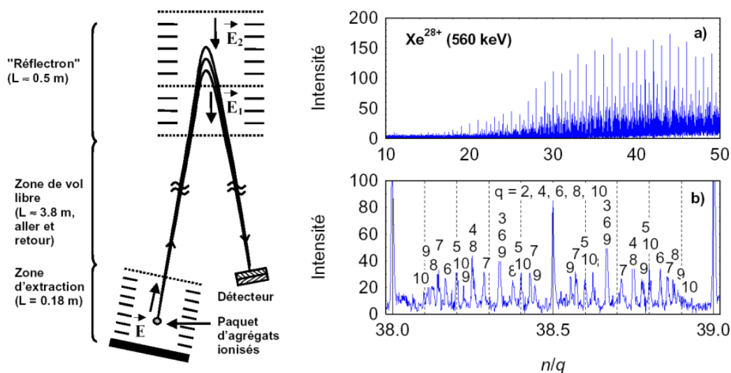
Figure 5 : A gauche : Schéma de principe du spectromètre de masse par temps de vol de type « reflectron ». A droite : a) Exemple d'un spectre de masse 29 obtenu avec ce spectromètre après la collision du jet d'agrégats neutres de sodium avec un faisceau d'ions lents de Xe^{28+} @ 560 keV ; b) détail du spectre a) mettant en évidence le pouvoir résolvant du spectromètre, qui permet d'identifier des agrégats multichargés jusqu'à un état de charge égal à 10.
