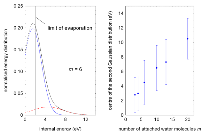
Figure 57 : A gauche, distribution d'énergie interne du système anionique \text{AMP}(\text{H}_2\text{O})_6^- , obtenu via la procédure d'ajustement des données sur la Figure 56. La contribution des deux fonctions gaussiennes est représentée ; les parties en pointillés dénotent la zone au le modèle d'ajustement n'est plus sensible. A droite, évolution de l'énergie centrale de la seconde distribution gaussienne en fonction de l'hydratation initiale (voir texte) ; les barres d'erreur symbolisent la largeur à mi-hauteur des distributions.
