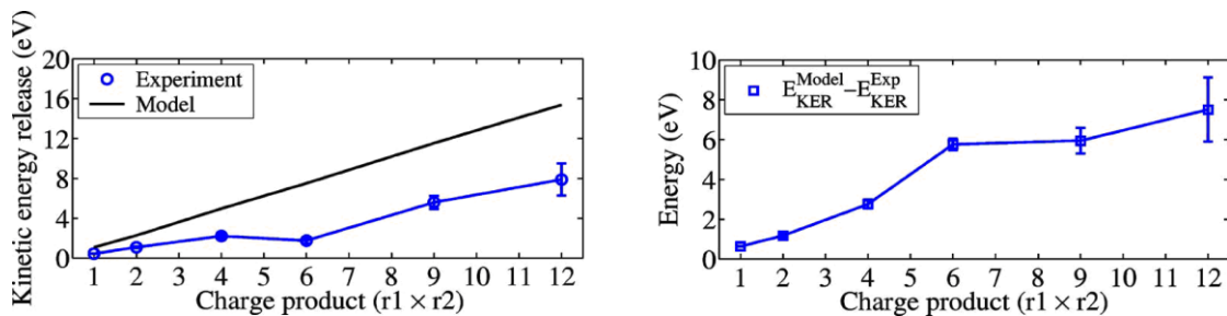
Figure 37 : Comparaison entre l'évolution expérimentale et théorique du KER en fonction du produit des charges des deux fragments, dus à une fission symétrique d'un dimère de C_{60} multiplement chargés.
