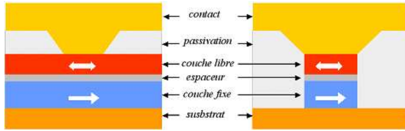
FIG. 2.1 : Deux types de dispositifs expérimentaux pour l'étude du transfert de spin. À gauche un contact ponctuel où est injecté le courant, une partie de la couche libre est excitée. À droite une structure confinée de type nano-pilier ; la couche dure est parfois partiellement gravée afin de limiter le couplage magnétostatique avec la couche libre.
