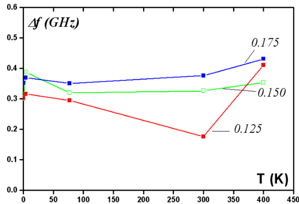
FIG. 5.24 : Variation de la largeur à mi-hauteur des pics de résonance en fonction de la température pour diverses valeurs de densité de courant (0.125, 0.15 et 0.175 10^{12} A/m 2 ). Les paramètres des calculs sont ceux du Permalloy : M_S=800 kA/m, A=10^{-11} J/m, \alpha=0.01 et \mathcal{P}=0.3 . La couche libre a pour dimensions 70*114*2.5 nm.
