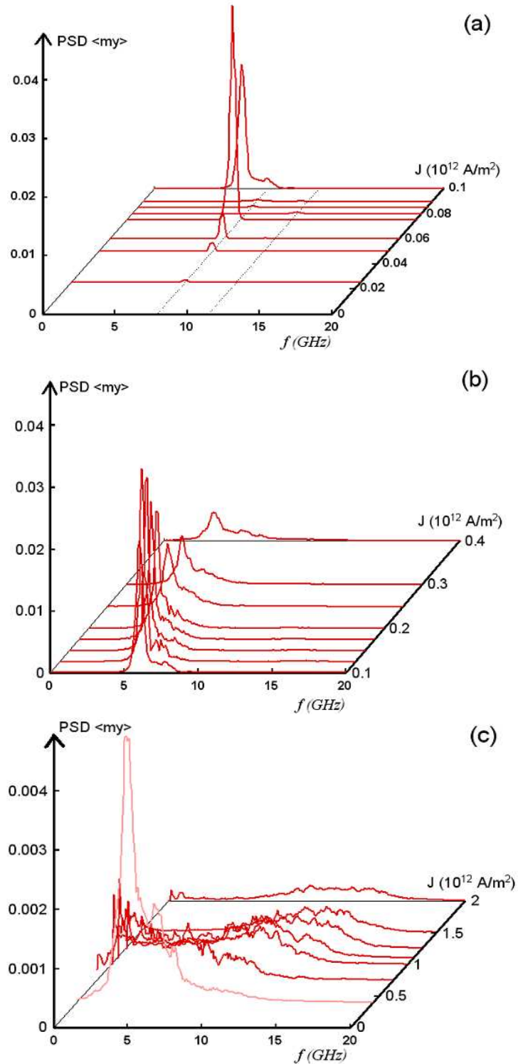
FIG. 5.13 : Densités spectrales de puissance de \langle m_y \rangle en fonction de la densité de courant injectée ( T=300 K). (a) pour les basses densités de courant ( J < 0.1 \cdot 10^{12} A/m 2 ), (b) régime de 'red-shift' pour les courants modérés ( J < 0.4 \cdot 10^{12} A/m 2 ) et (c) régime de 'blue-shift' des fréquences pour les forts courants ( J > 0.4 \cdot 10^{12} A/m 2 ). Le champ appliqué de 3 \cdot H_K . Les paramètres des calculs sont ceux du Permalloy : M_S = 800 kA/m, A = 10^{-11} J/m, \alpha = 0.01 et P = 0.3 . La couche libre a pour dimensions 70 \cdot 114 \cdot 2.5 nm.
