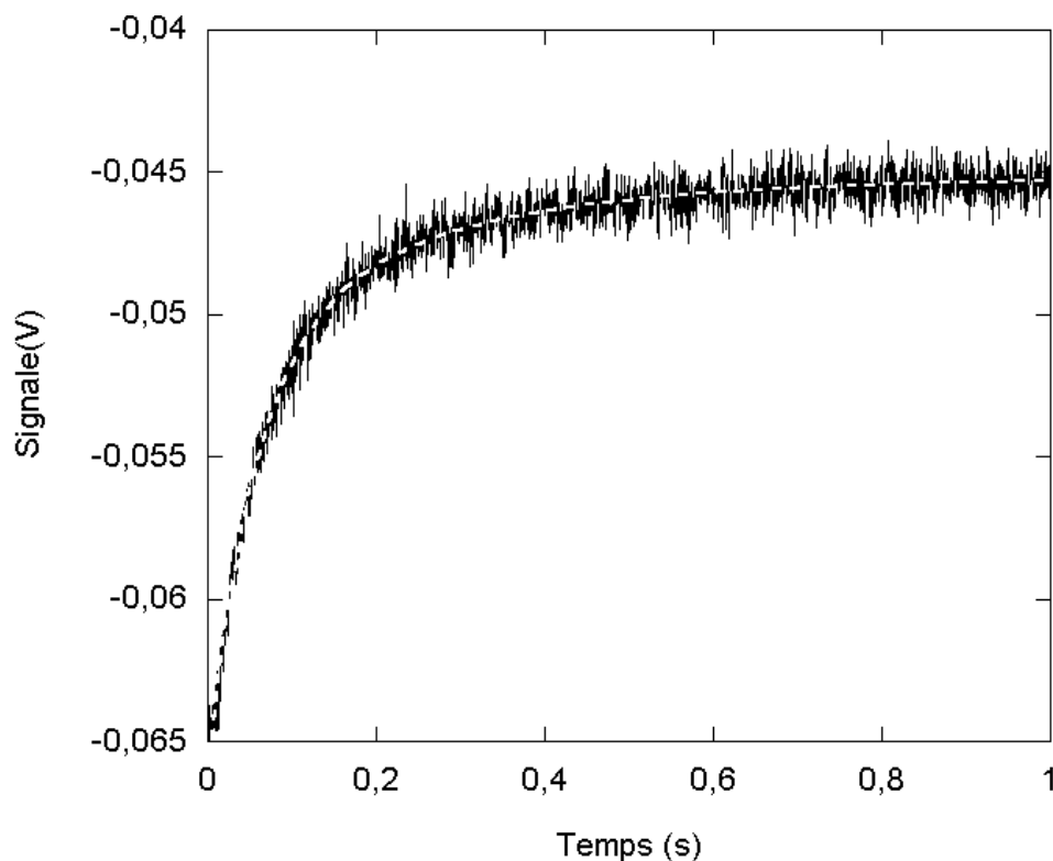
Figure 5.8 : Cinétique de l'association de la phthalocyanine l'aluminium disulfonée aux LDL : Exemple de signal de fluorescence enregistré après le mélange de la phthalocyanine ( 4,4 \times 10^{-8} M) avec les LDL ( 1,5 \times 10^{-7} M). Le meilleur ajustement bi-exponentiel est superposé au signal.
