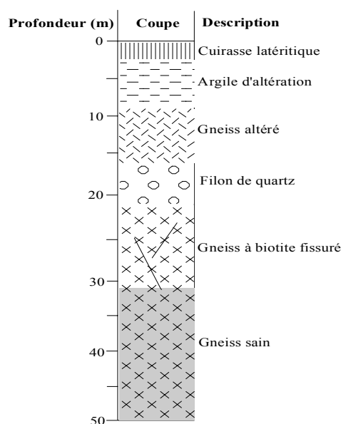
Figure 13 : Coupe lithostratigraphique du forage de Béléfongou.
