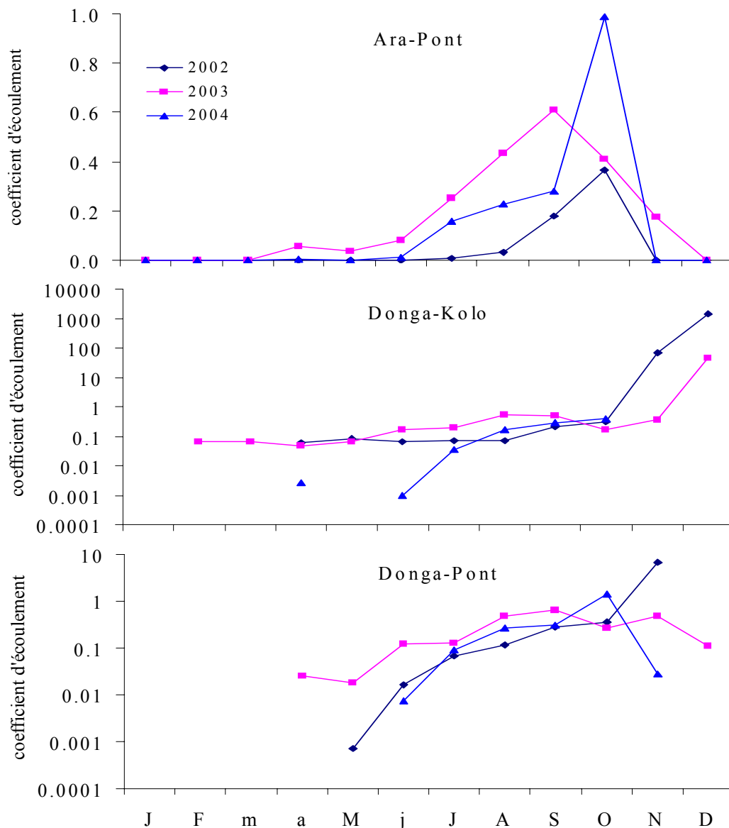
Figure 46 : Coefficient d'écoulement \alpha ( L_e/L_p ) mensuels sur les 3 bassins pour les années 2002, 2003 et 2004 ; L_p = lame précipitée (mm) et L_e = lame écoulée (mm).
