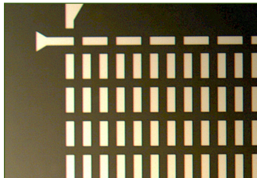
FIG. 5.8 – Vue partielle d’une série après gravure et délaquage de la résine. Sur le fond (partie foncée) le substrat est couvert par une couche mince de MgO.
