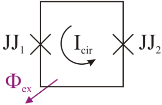
FIG. 2.5 – SQUID dc constitué par deux jonctions Josephson dans une boucle supraconductrice. En présence d'un flux magnétique externe \Phi_{ex} la boucle est traversée par un courant circulaire I_{cir} . Dans cette condition I_{J1} = -I_{J2} . L'inductance des lignes a été négligée dans l'hypothèse où elle est \ll L_J .
