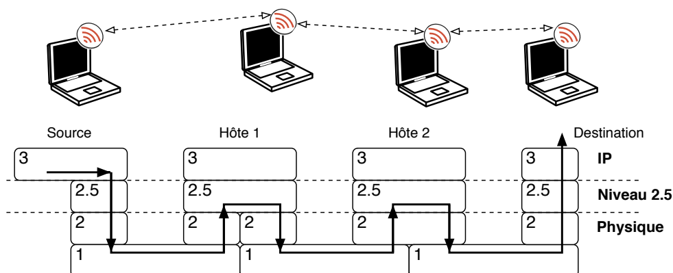
FIG. 3.6 – Utilisation d'un niveau 2.5 pour l'acheminement de données
