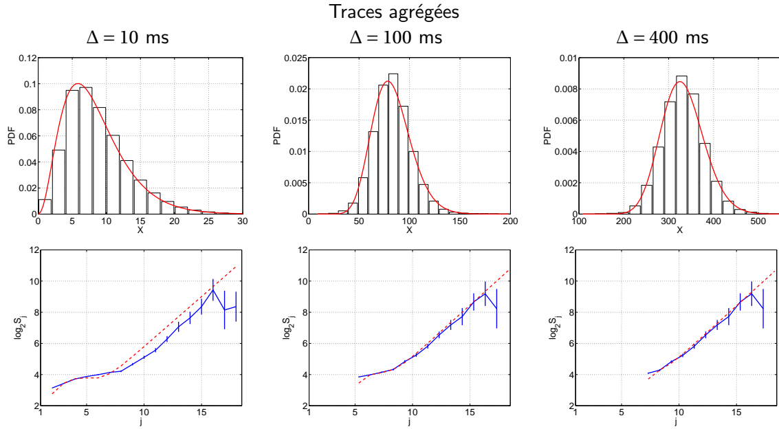
Fig. 4.2: Analyse de la trace AuckIV. Ajustements des histogrammes empiriques par une loi Gamma( \alpha, \beta ) (première ligne) et des covariances par un processus FARIMA( \phi, d, \theta ) (deuxième ligne).
