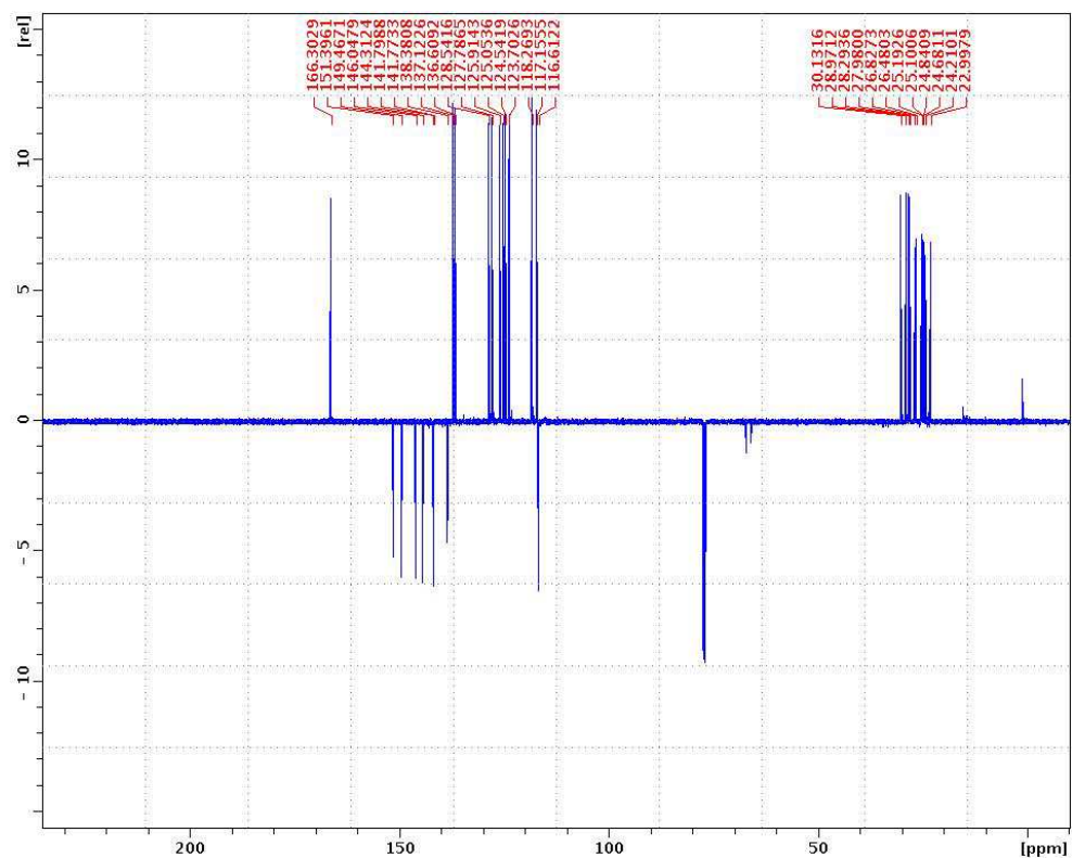
Figure 2 : Spectre de RMN du carbone 13 ( \text{CDCl}_3 ) du germylène 32b
