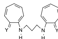
24a Y = N- i -Pr 24b Y = O
