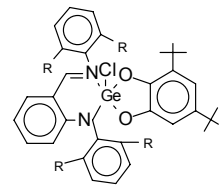
35a R= Me 35b R= i -Pr
