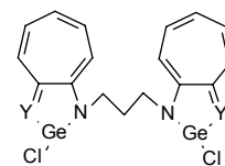
26a, Y = N- i -Pr 26b, Y = O
