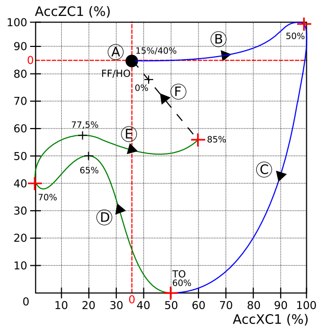
FIG. 3.25 – Cyclogramme des variations de l'accélération antéro-postérieure en fonction des variations de l'accélération craniale-caudale pour un capteur placé sur le tibia. En bleu est la phase de support, en vert la phase de vol, les lettres correspondant à diverses phases du cycle de marche (A : Midswing, B : Terminal stance, C : Preswing, D : Initial swing, E : Midswing, F1 : Terminal swing, F2 : Loading response)
