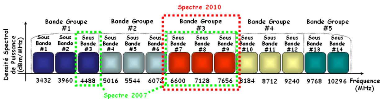
Figure IV.11 : Diagramme d’allocation des sous-bandes MB-OFDM pour les communications ULB en Europe, dans sa définition actuelle en 2007, et future en 2010.
