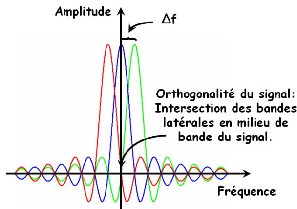
Figure II.3 : Division du spectre en SB ( N_{SP}=3 ) et notion d'orthogonalité entre les sous-porteuses pour les systèmes OFDM.
