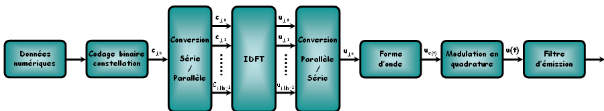
Figure II.5 : Schéma de principe d'un émetteur multi-porteuses OFDM.
