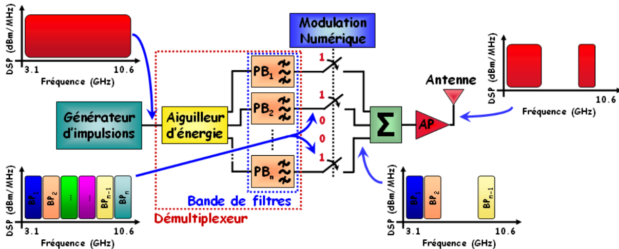
Figure II.16: Schéma de principe de l'émetteur MB-OOK, exemple de transmission.
