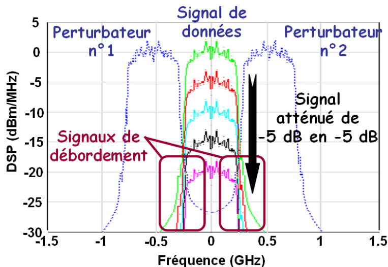
Figure III.4 : DSP du signal ULB-OFDM transmis et des sous-bandes adjacentes.
