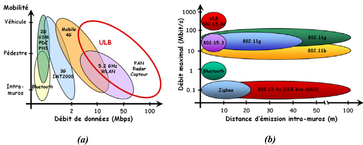
Figure I.2 : Positionnement des systèmes ULB par rapport aux systèmes existants en terme de débit et de mobilité (a), en terme de débit et de portée (b).
