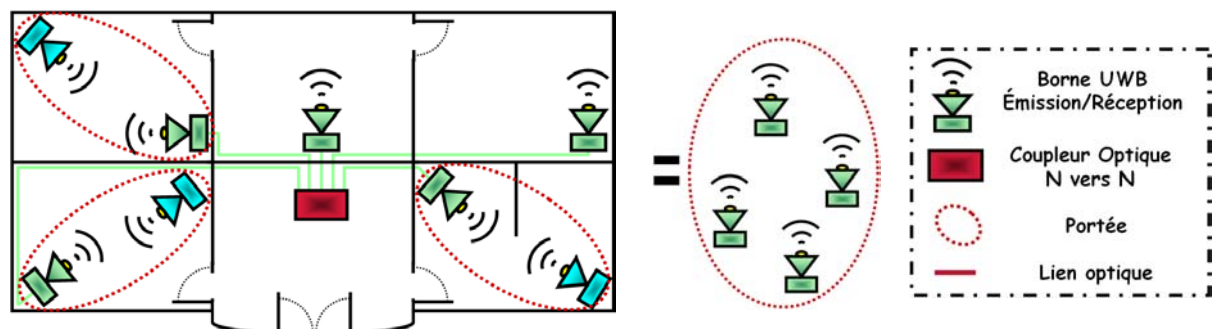
Figure I.20 : Schéma d'un réseau hybride radio-filaire avec liens multipoints à multipoints en radio sur fibre basé sur un coupleur N vers N.
