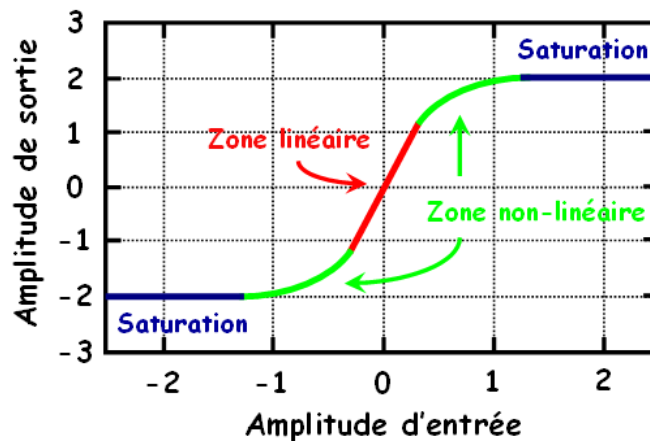
Figure III.5 : Réponse en tension typique d'un amplificateur.
