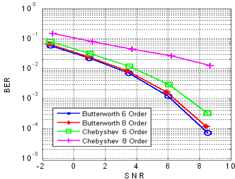
Figure III.28 : Variation du BER en fonction du rapport SNR pour les différents types et ordres de filtrages.
