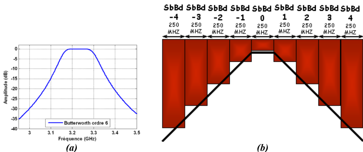
Figure III.20 : Exemple de fonction de transfert d'un filtre Butterworth d'ordre 6 (a), et illustration de son découpage en sous-bandes SsBd (b).
