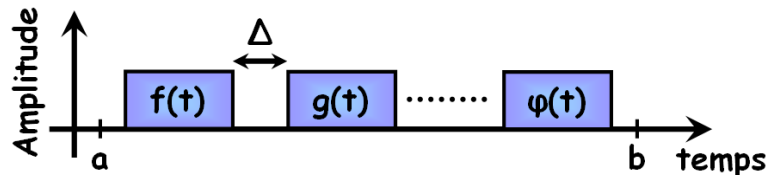
Figure II.2 : Base orthogonale dans le domaine temporel à l'aide de fonctions portes.
