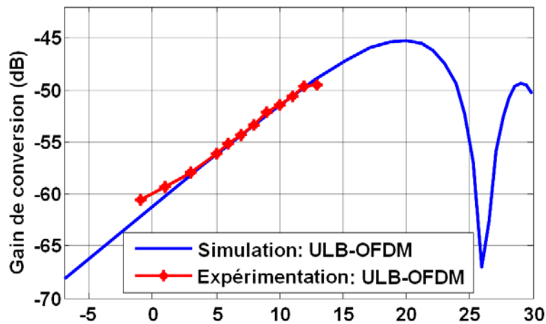
Figure IV.24 : Comparaison du gain de conversion optique G_{CV_{Opt}} simulé et mesuré, en fonction de la puissance du signal d'OL.
