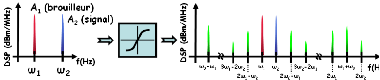
Figure A2.1 : Génération de produits d'IM à partir de deux signaux fondamentaux traversant une fonction non-linéaire.
