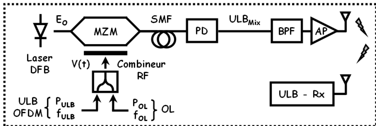
Figure IV.17 : Lien RoF pour la conversion de fréquence de signaux ULB-OFDM par voie optique avec un modulateur externe MZM.
