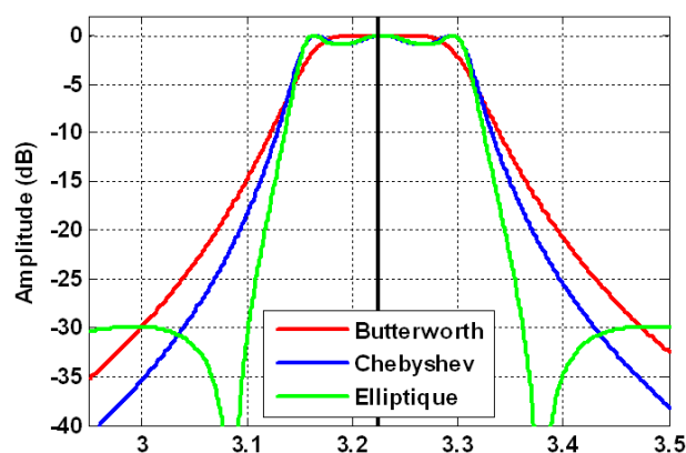
Figure III.17 : Exemple de fonction de transfert pour les 3 types de filtres, de fréquence centrale F_c = 3230 MHz et d'ordre 6.
