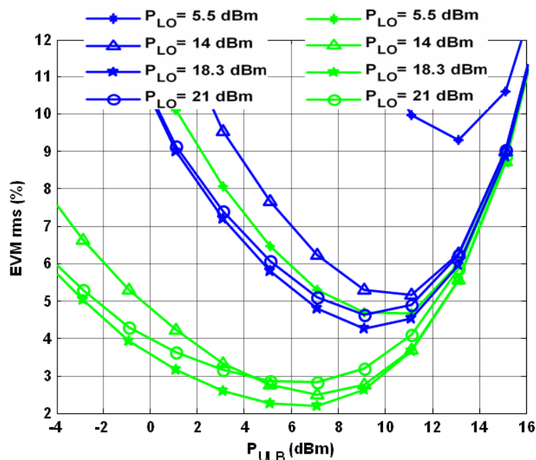
Figure IV.22 : Variation de l'EVM en fonction de la puissance P_{ULB} aux points de polarisations MIN-T et MAX-T, pour différentes valeurs de puissances P_{OL} .
