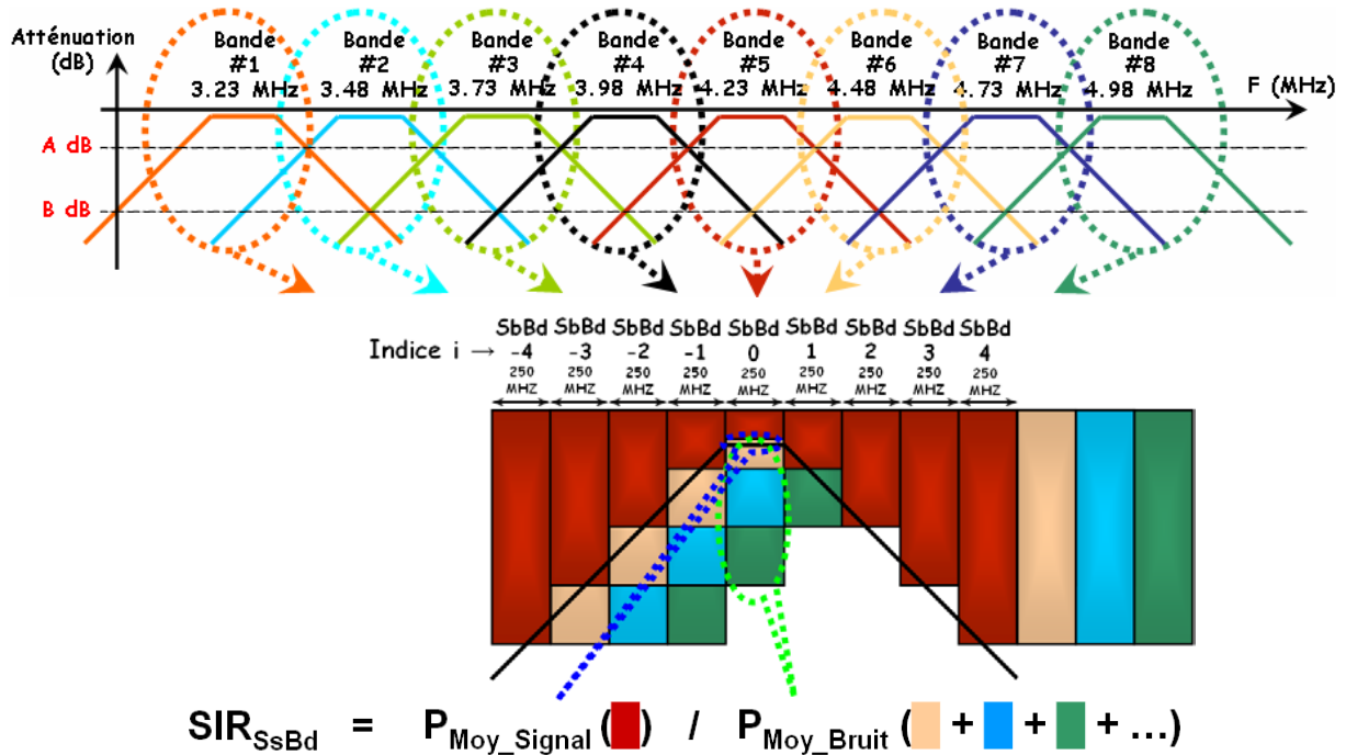
Figure III.21 : Illustration du processus de calcul du rapport SIR_{SsBd} .
