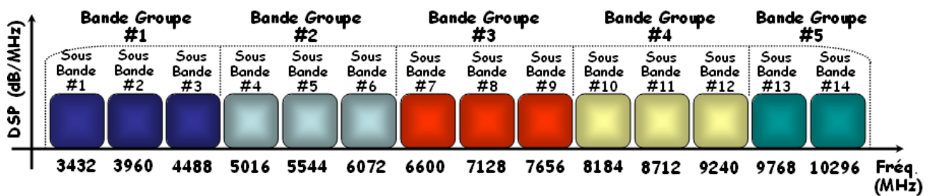
Figure I.16 : Diagramme d’allocation des 14 sous-bandes pour les communications ULB MB-OFDM.
