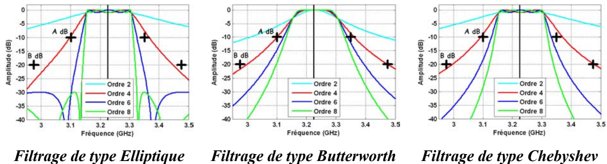
Figure III.19 : Fonction de transfert pour les 3 types de filtres, de BP = 150 MHz de fréquence centrale F_C = 3230 MHz.
