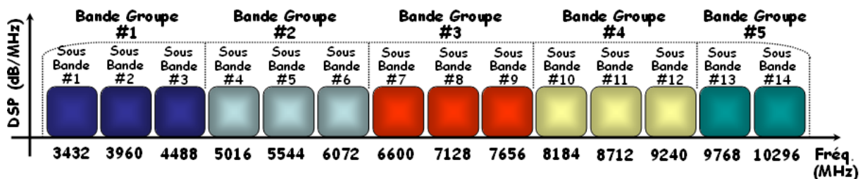
Figure II.8 : Découpage fréquentiel de la bande ULB comprise entre 3,1 et 10,6 GHz en 14 SB regroupées en 5 groupes de bandes.
