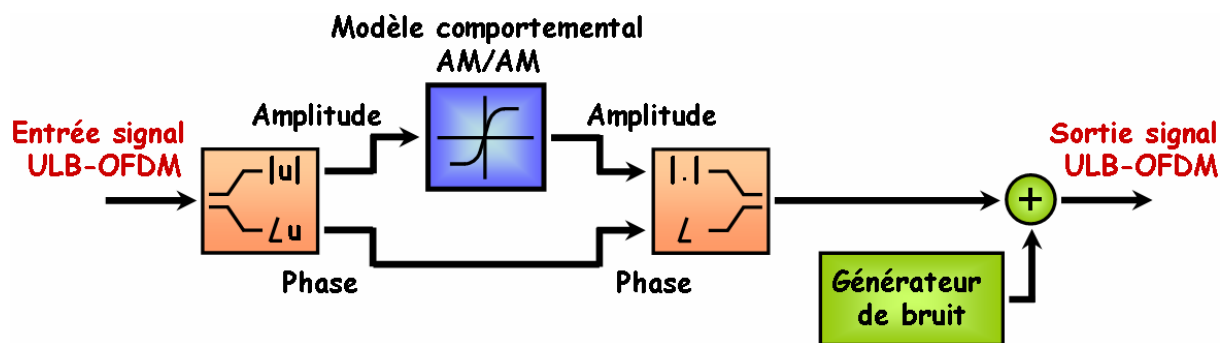
Figure IV.9 : Modèle comportemental des systèmes de transmission ULB sur fibre.
