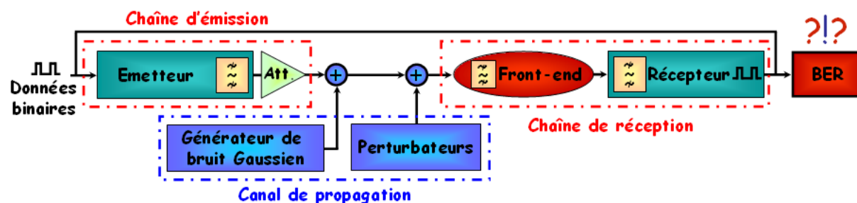
Figure III.2: Chaîne de transmission ULB-OFDM et front-end RF de réception.
