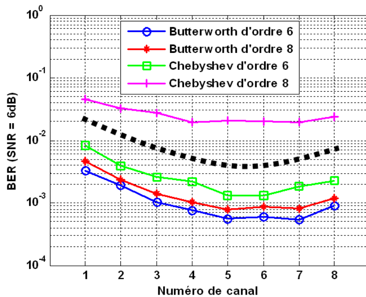
Figure III.26 : Variation du BER en fonction du numéro de canal avec un SNR de 6 dB pour des filtres Butterworth et Chebyshev.
