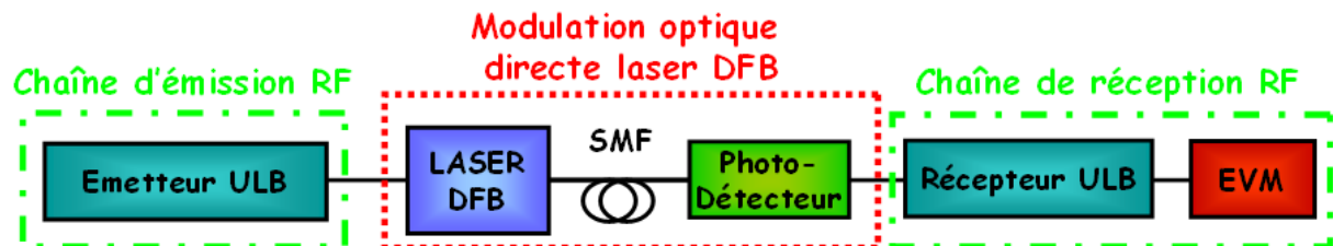
Figure IV.4 : Chaîne de transmission ULB sur fibre avec une transmission directe (laser DFB directement modulé).
