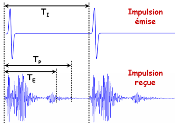
Figure II.21 : Réponse impulsionnelle typique du canal de propagation ULB par rapport au signal émis.
