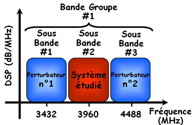
Figure III.3 : Disposition du système étudié par rapport aux perturbateurs dans le groupe de bande GB#1.
