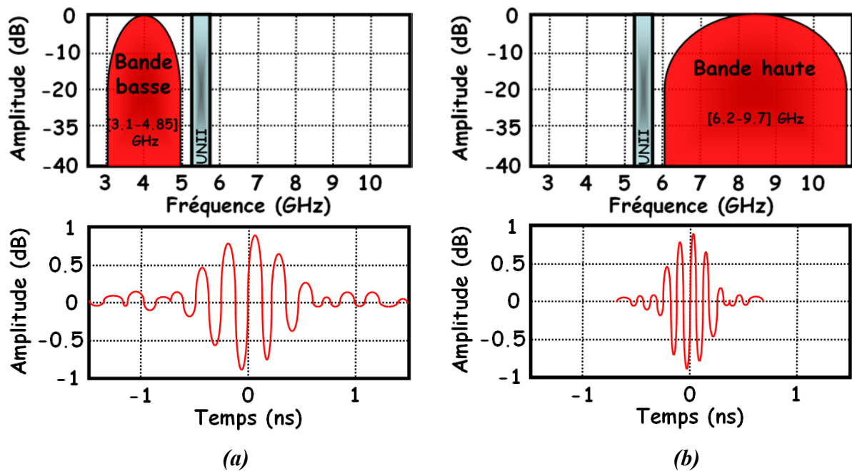
Figure I.14 : Spectres et formes d’ondes temporelles IR-ULB pour la bande basse (a) et haute (b).
