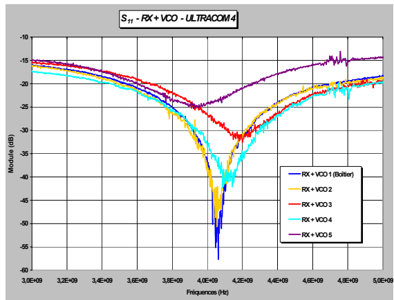
(b) Paramètre S_{11} mesuré en entrée.
