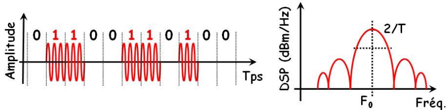
Figure II.15 : Modulation OOK et spectre fréquentiel associé.
