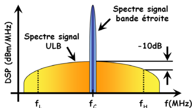
Figure I.1 : DSP pour un système ULB et un système à bande étroite.
