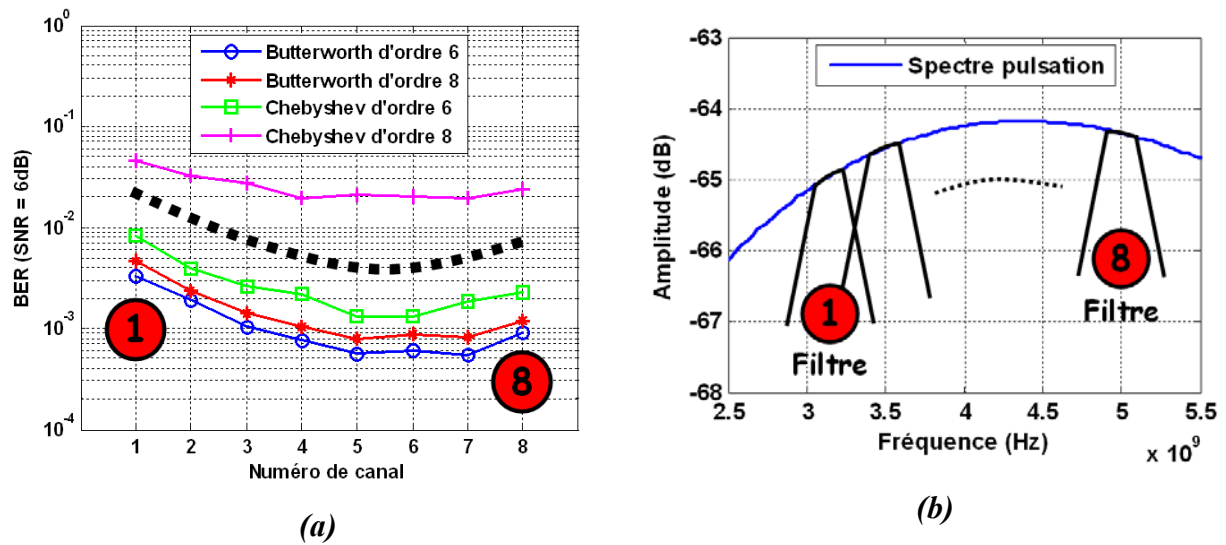
Figure III.27 : BER en fonction du numéro de canal (a) en opposition au spectre en fréquence du signal d'entrée (b).
