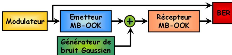
Figure III.25 : Schéma synoptique de la chaîne de transmission MB-OOK.
