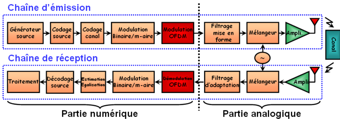
Figure II.4 : Schéma synoptique d'une chaîne d'émission/réception OFDM.
