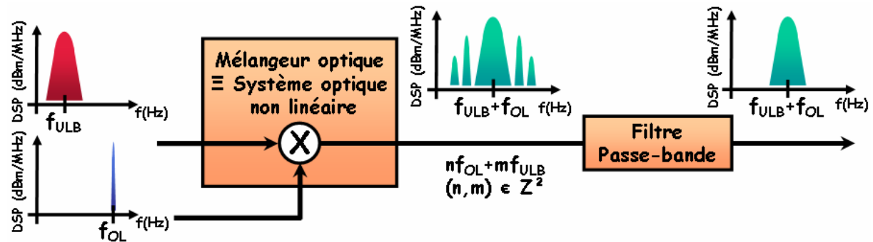
Figure I.21 : Schéma de principe d'un mélangeur électro-optique, cas d'une conversion haute fréquence.
