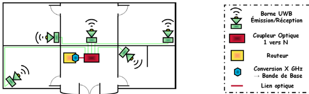
Figure I.19 : Schéma d'un réseau hybride radio-optique avec liens point-à-multipoints RoF basé sur un coupleur 1 vers N.
