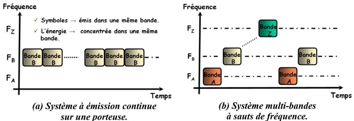
Figure I.11 : Schéma temporel d’occupation des bandes pour un système de transmission mono et multi-bandes.
