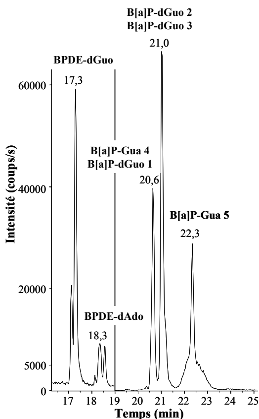
Figure 25 : Chromatogramme obtenu pour l'injection de 500 fmoles de chaque adduit de l'ADN. Chaque pic correspond à la superposition des transitions utilisées pour la détection de l'adduit concerné.
