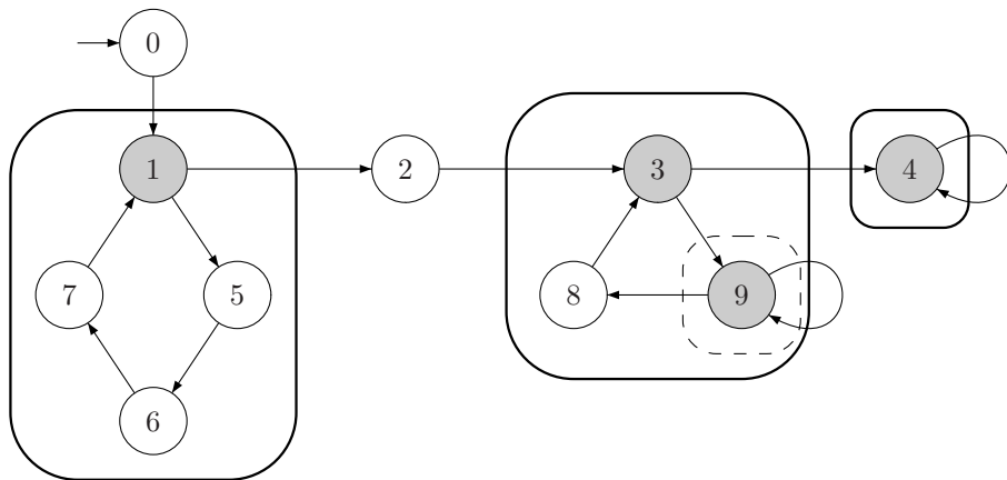
FIG. 2.4 – Un automate et ses CFC et sCFC
