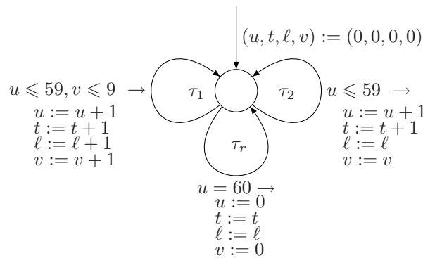
FIG. 7.7 – La chaudière deuxième version
