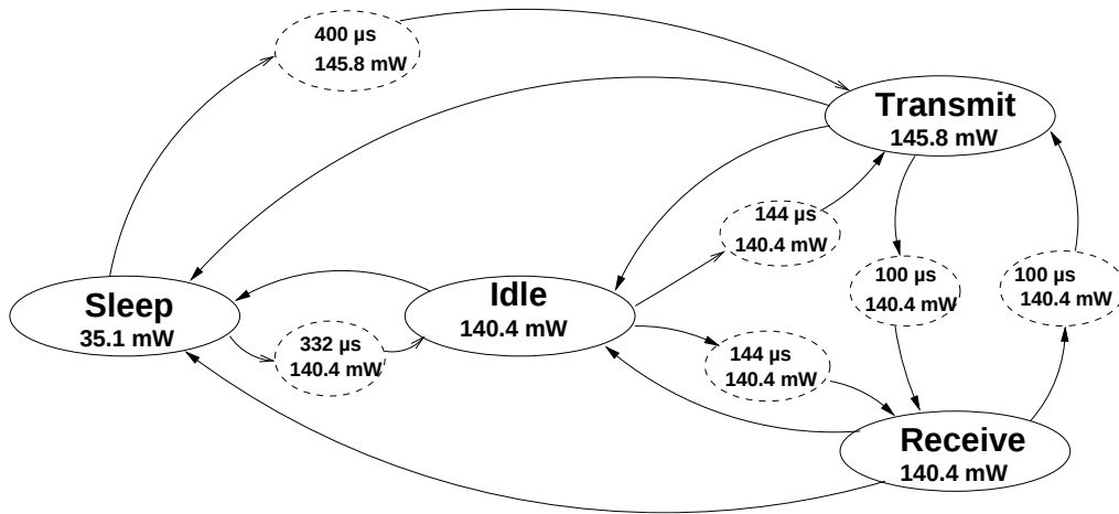
FIG. 9.7 – Automate modélisant la consommation d'une radio ([SMMM06])
