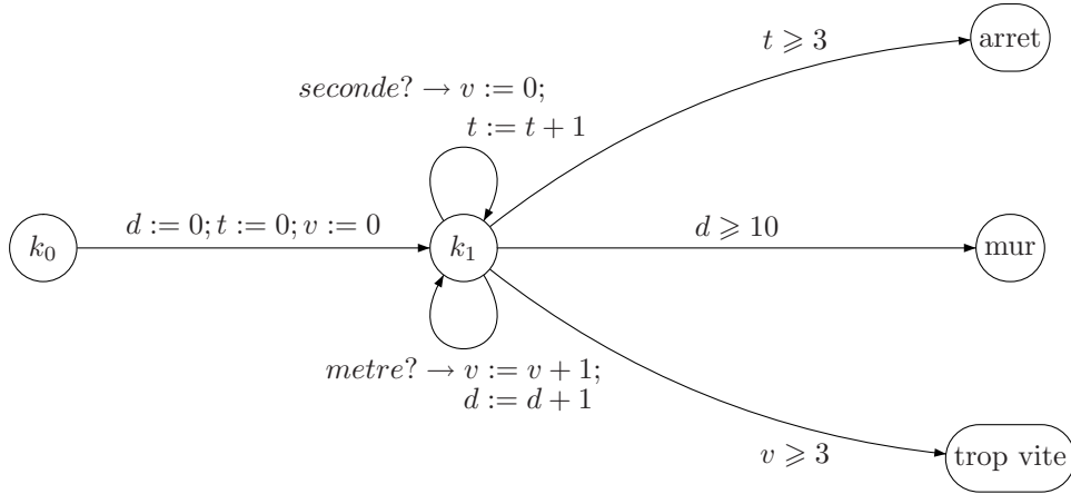
FIG. 4.5 – Automate interprété avec entrées booléennes modélisant une voiture
