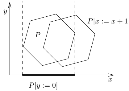
FIG. 2.10 – Image d'un polyèdre par une action affine
