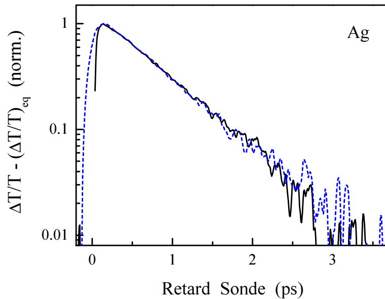
FIG. 2.13: Evolution temporelle du changement de transmission \Delta T/T normalisé mesuré dans des nanoparticules d'argent de diamètre moyen D = 1.5 nm dispersées dans une matrice d'alumine. La sonde est hors résonance ( \hbar\omega_s = 1.5 eV ) et la pompe dans l'infrarouge ( \hbar\omega_p = 1.5 eV ) ce qui correspond à une élévation de température électronique \Delta T_e \approx 1700 K (trait plein) ou dans le bleu ( \hbar\omega_p = 3 eV ), correspondant à \Delta T_e \approx 2500 K (tirets).
