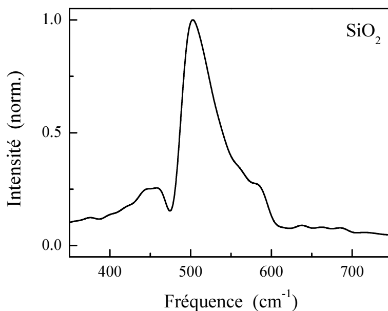
FIG. 3.12: Transformée de Fourier FFT du signal temporel pour un temps de coupure à 88 fs.
