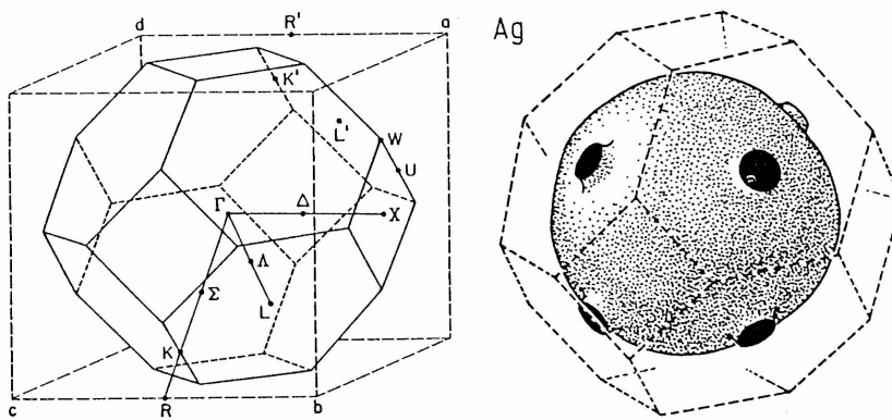
(b) Structure de bandes pour des électrons libres d'un réseau cfc projetée sur différentes directions de la première zone de Brillouin. Source : [16].
