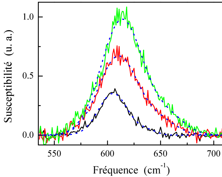
FIG. 3.20: Modes D_2 extraits du spectre Raman réduit après soustraction d'un fond polynomial (traits pleins) et leurs ajustements par des gaussiennes (pointillés) pour des densités \rho = 2.20, 2.43 et 2.63 \text{ g.cm}^{-3} . L'amplitude du mode D_2 croît avec la densité.
