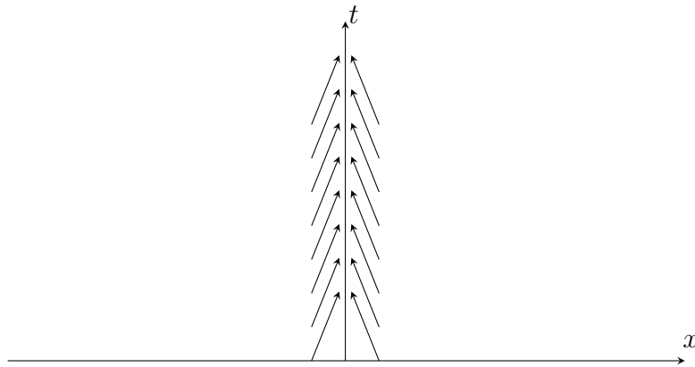
Représentation du champ de vecteurs \partial_t + a(t, x)\partial_x au voisinage de l'interface pour un cas compressif
