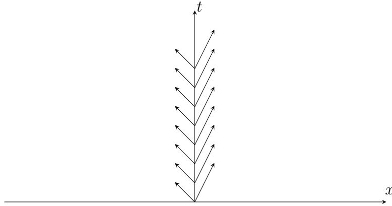
Représentation du champ de vecteurs \partial_t + a(t, x)\partial_x au voisinage de l'interface pour un cas expansif
