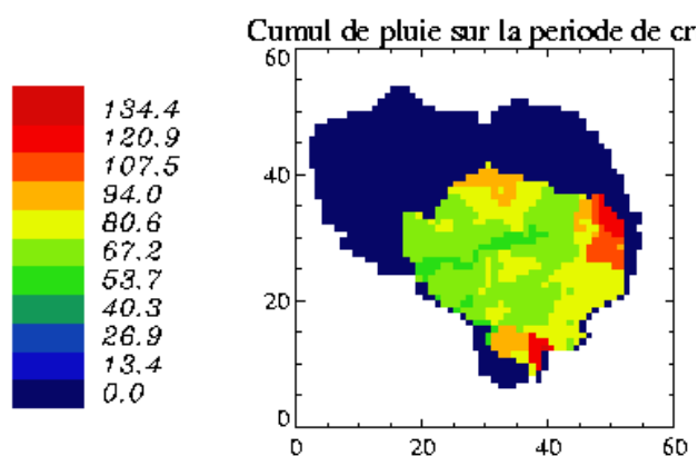
FIG. 5.34 – Cumul de précipitations lors de la crue 0001-2
