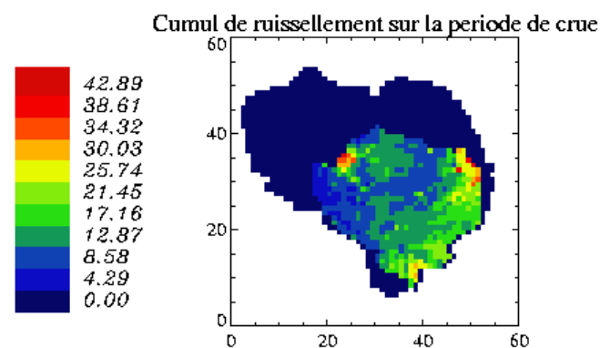
FIG. 5.23 – Cumul de ruissellement lors de la crue 9900-2
