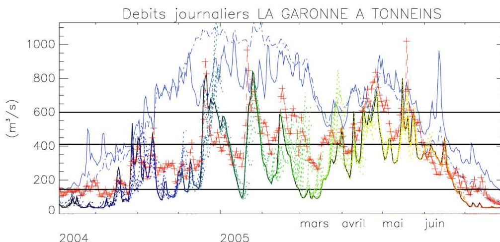
FIG. 5.3 – Débits du 4 sept 2004 au 31 juil 2005 pour la Garonne à Tonneins. Croix rouges : observations; Trait noir continu : analyse SIM; Traits pointillés : chaque jour, moyenne de l'ensemble à 10 jours; Traits bleus pointillés : climatologie observée et climatologie SIM 1981-2004; Traits horizontaux noirs : valeur des seuils utilisés pour l'analyse statistique.
