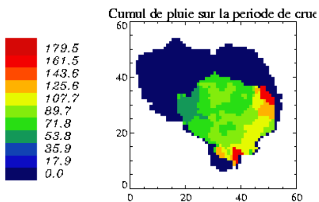
FIG. 5.22 – Cumul de précipitations lors de la crue 9900-2
