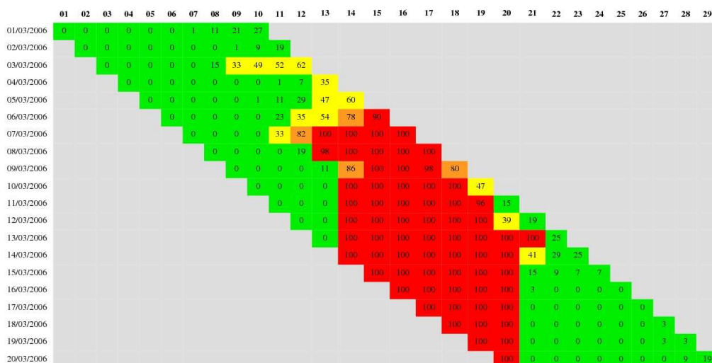
FIG. 2.24 – Tableau d'alerte pour la Seine à Paris, Mars 2006, pour le dépassement du seuil 700 \text{ m}^3 \text{ s}^{-1} . Probabilité < 30 % : vert ; 30 %-70 % : jaune ; 70 %-90 % : orange, > 90 % : rouge.
