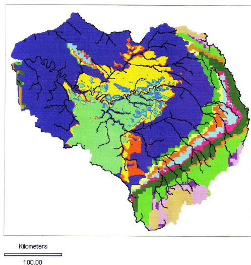
FIG. 1.5 – Carte géologique simplifiée ([GOMEZ 2002])
