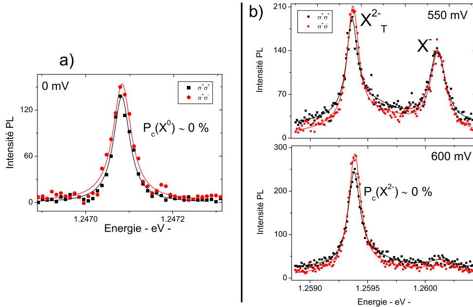
FIG. 3.4: Mise en évidence de la faible polarisation circulaire (a) d'un exciton neutre pour une excitation à 1.31 eV et (b) du complexe X^{2-} pour une excitation à 1.32 eV. On peut noter sur (b) que le trion X^- est lui aussi très peu polarisé, fondamentalement pour la même raison que X^{2-} à cette tension.
