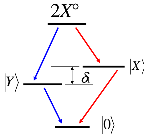
FIG. 1.13: Cascade radiative du biexciton, montrant la corrélation de polarisation due aux règles de conservation du moment angulaire.
