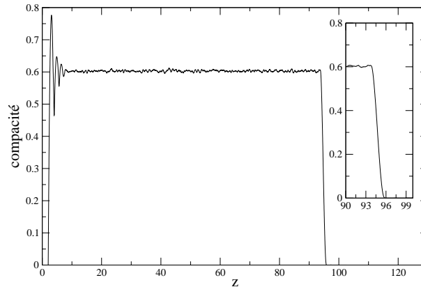
Figure 3.2: Exemple de profil de compacité d'un empilement généré via l'algorithme de Powell. L'encart montre que la compacité décroît jusqu'à une valeur nulle sur une hauteur de l'ordre de deux diamètres de grains.
