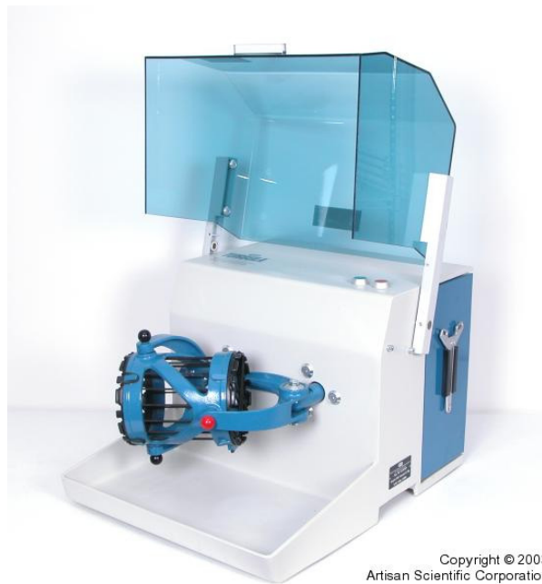
Figure 1.13: Photographie d'un turbula (d'après une documentation technique de Artisan Scientific).
