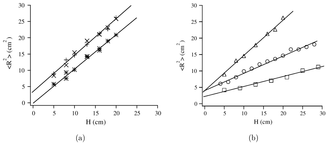
Figure 1.26: Résultats expérimentaux d'après Ippolito et al. (2000). (a) Évolution de la variance des positions dans la direction perpendiculaire à l'écoulement en fonction de la hauteur H pour D = 16 mm et (+) d = 0,7 mm, (\times) d = 1 mm et (*) d = 2 mm. (b) Influence de la taille des particules constituant le milieu poreux. \langle R^2 \rangle en fonction de H pour (\square) D = 6 mm, (\circ) D = 10 mm et (\triangle) D = 16 mm.
