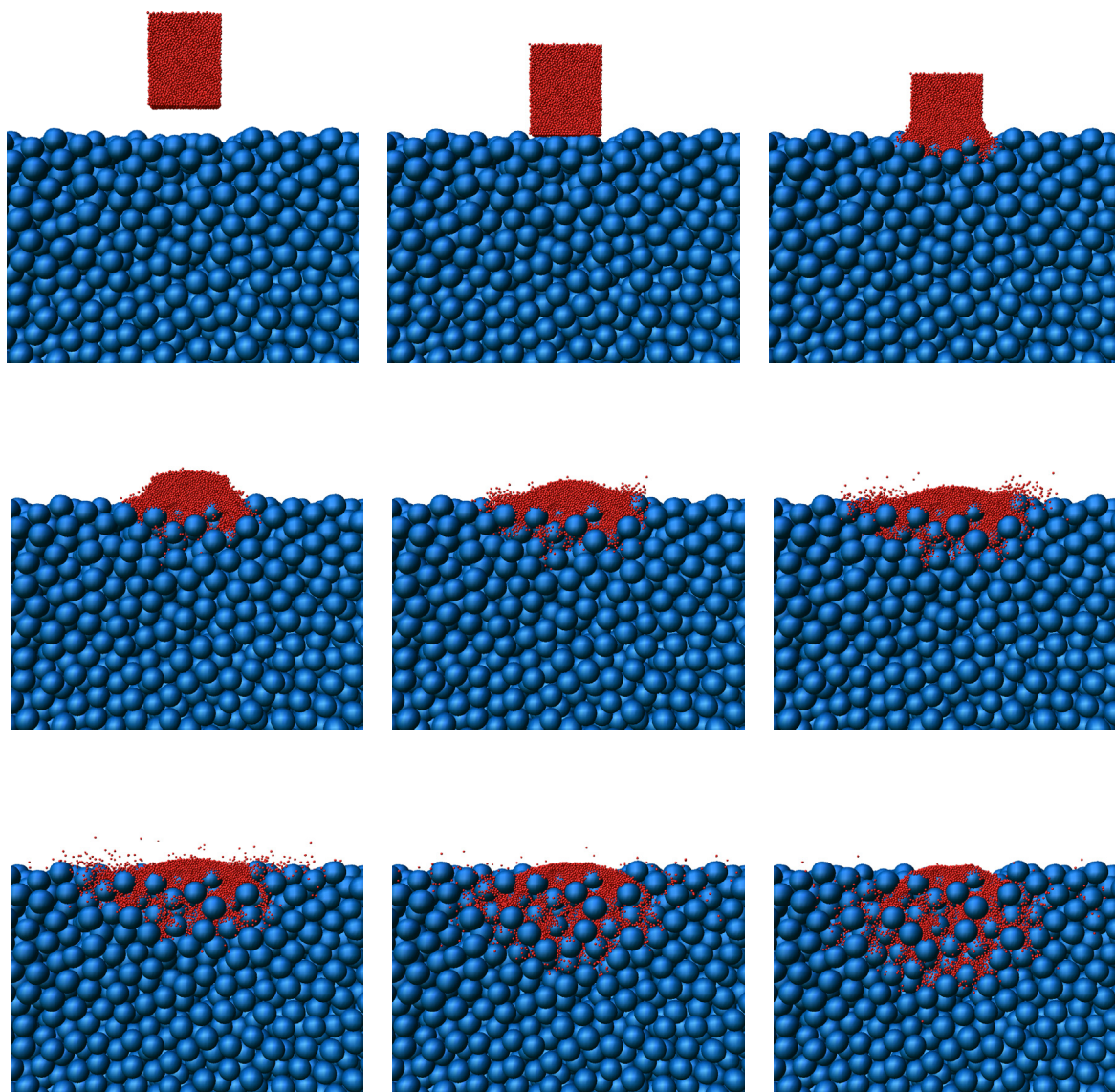
Figure 4.1: Série de clichés pris à différents instants illustrant la pénétration et l'écoulement de particules dans un milieu poreux via l'utilisation de la modélisation numérique. Pour permettre une visualisation convenable, seulement la moitié du milieu poreux est représentée. Ces illustrations ont été obtenues par la méthode de dynamique moléculaire de sphères molles.
