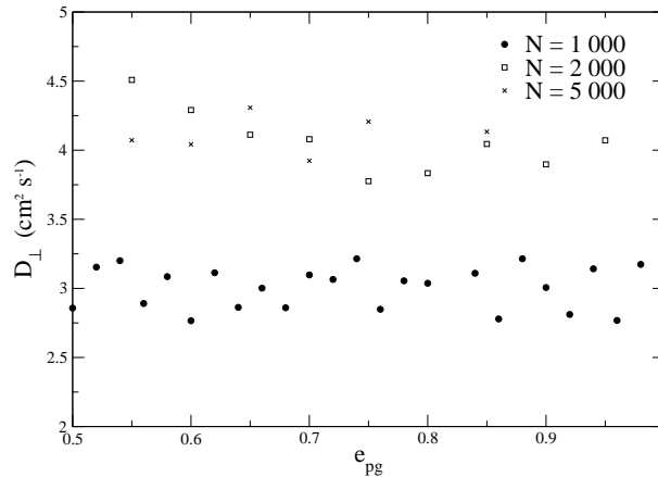
Figure 4.33: Évolution du coefficient de dispersion D_{\perp} en fonction du coefficient de restitution e_{pg} pour N = 1\,000 , N = 2\,000 et N = 5\,000 . Ces résultats ont été obtenus par la méthode MD avec H/D = 14 et e_{pp} = 0,99 .
