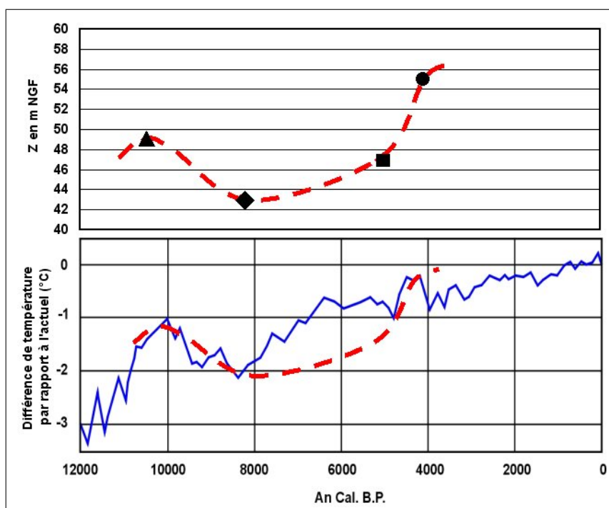
FIG. 2.42 – Corrélation : hauteurs des grès de Coudures et courbe paléoclimatique
