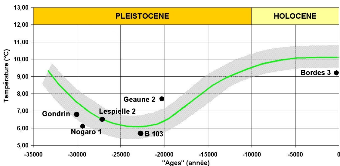
FIG. 2.6 – Evolution paléoclimatique au sud du Bassin Aquitain [BLAVOUX et al. (1993)] - Températures déduites à partir des teneurs en gaz rares des eaux
