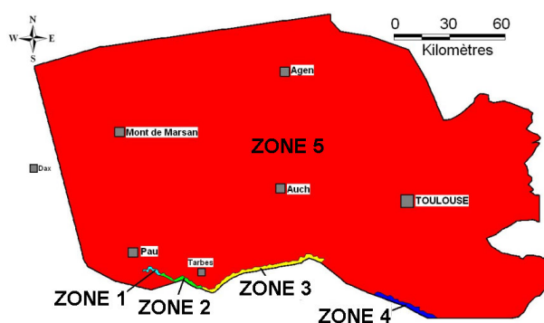
FIG. 3.60 – Zones de recharge potentielle pour un modèle d'évolution paléoclimatique
