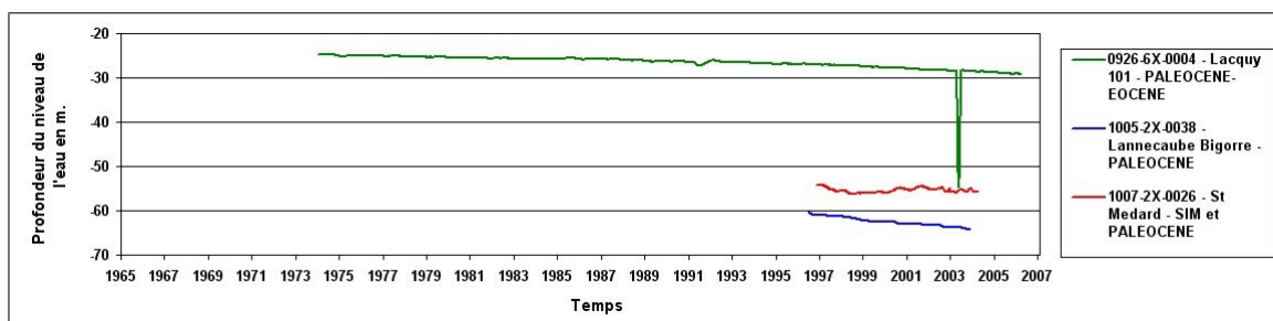
FIG. 1.52 – Evolution de la profondeur du niveau de l’eau pour les forages ne subissant pas ou peu les effets des stockages de gaz : autres Aquifères
