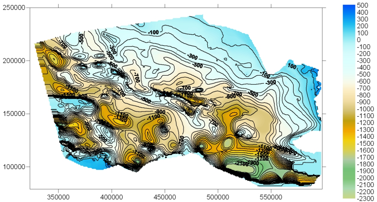
TOIT DES SABLES EOCENES
