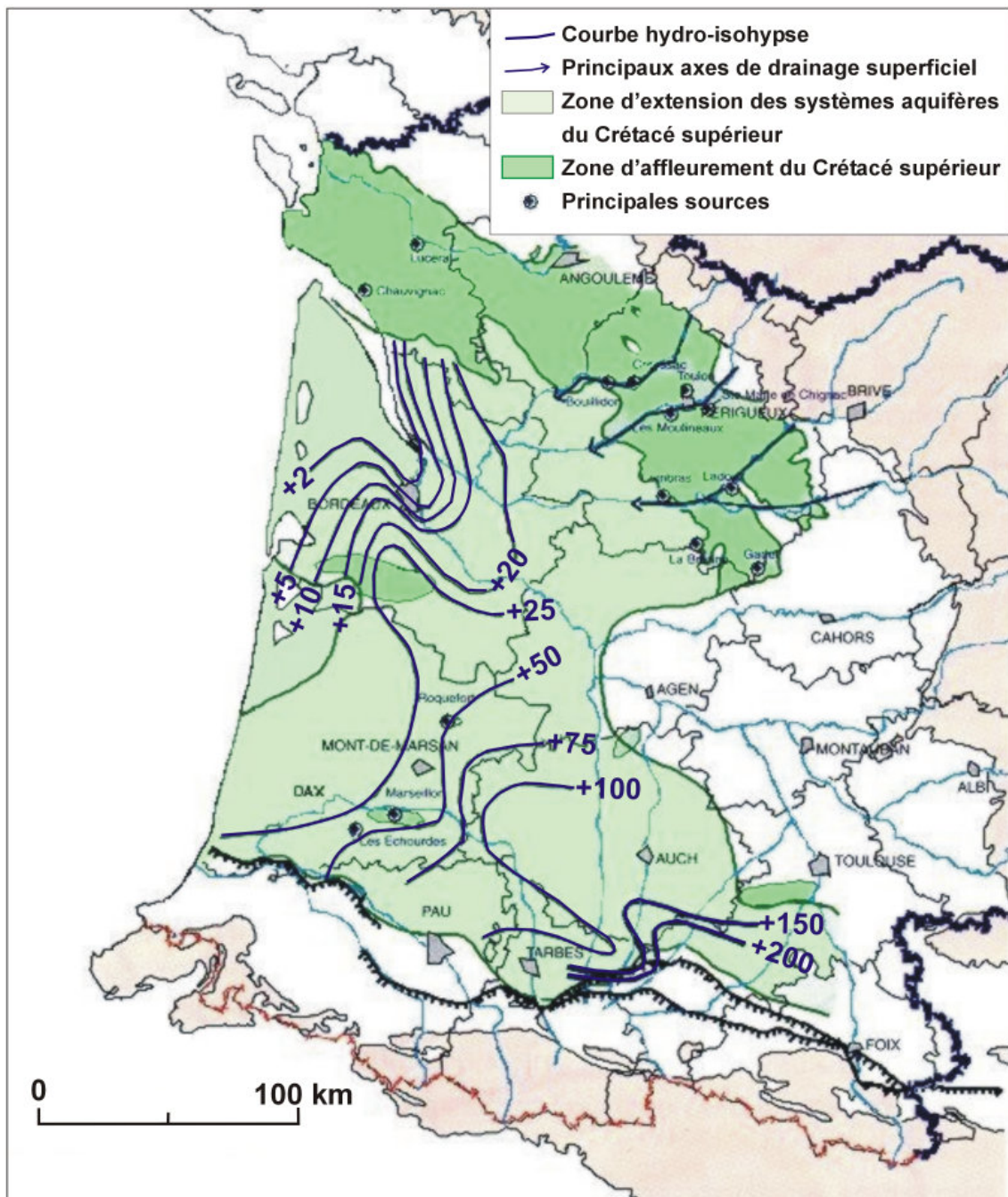
FIG. 1.38 – Esquisse piézométrique de la nappe du Crétacé supérieur [d’après MAUROUX et DANNEVILLE (1996)]
