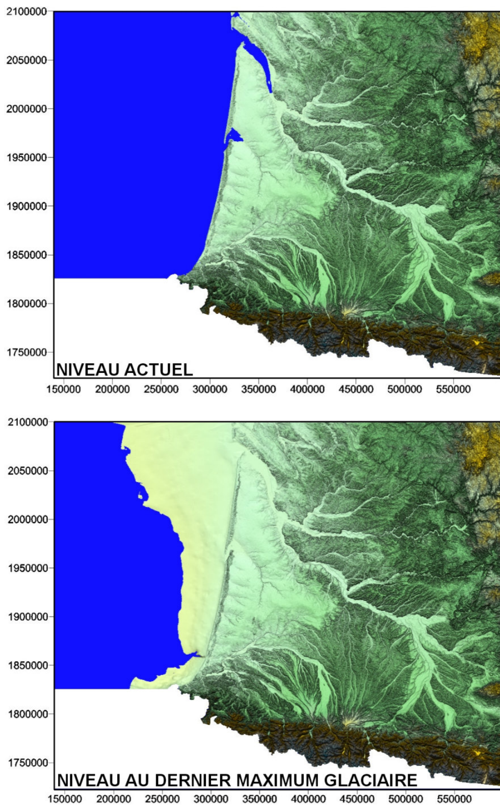
FIG. 2.14 – Evolution du trait de côte du golfe de Gascogne entre le Dernier Maximum Glaciaire et l'actuel
