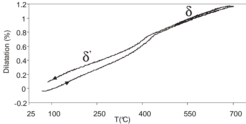
Figure III.35. : Courbe de dilatométrie de Pb_2BiV_{0.75}P_{0.25}O_6 montrant la transition \delta' \leftrightarrow \delta
