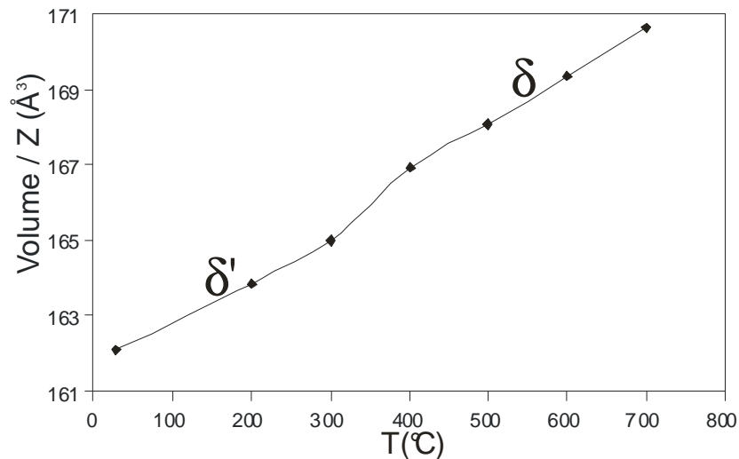
Figure III.34. : Évolution du volume formulaire ( \text{\AA}^3 ) en fonction de la température de Pb_2BiV_{0.75}P_{0.25}O_6
