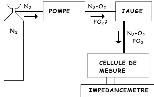
Figure IV.3. : Schéma du montage expérimental
