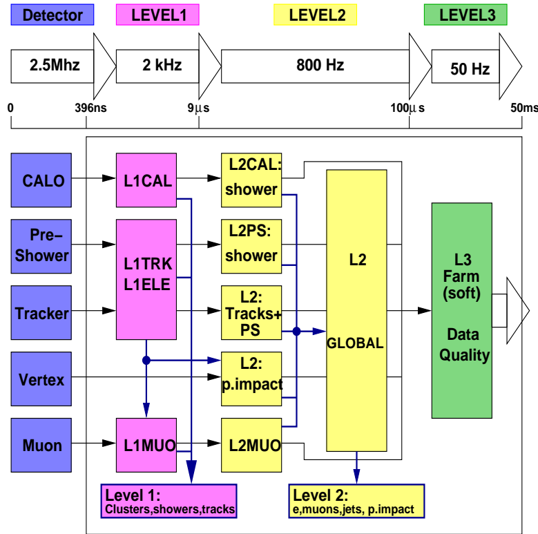
FIG. 4.1 – Vue schématique du système de déclenchement à D\bar{O} .
