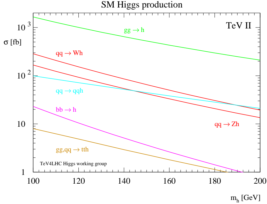
FIG. 1.3 – Sections efficaces de productions (fb) du boson de Higgs au Tevatron ( \sqrt{s} = 1.96 TeV) pour les processus de production les plus importants en fonction de la masse du boson de Higgs [17].
