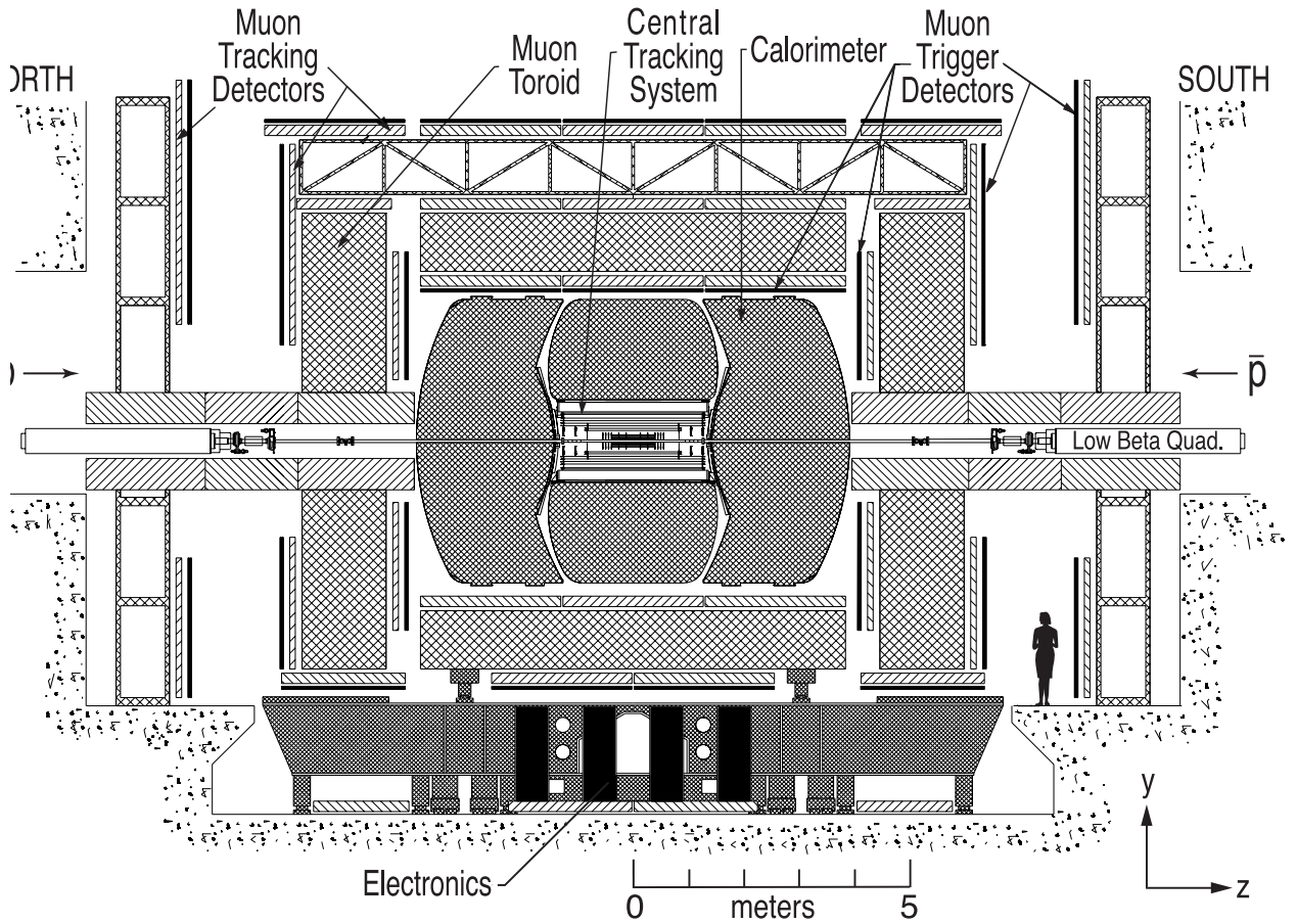
FIG. 3.4 – Le détecteur DØ au Run II.
