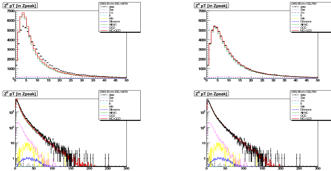
FIG. 2.5 – Distributions du p_T du boson Z dans les données (points) et la simulation (ALPGEN, histogramme) pour les événements Z(ee)+jets avant (gauche) et après (droite) pondération du p_{TZ} .
