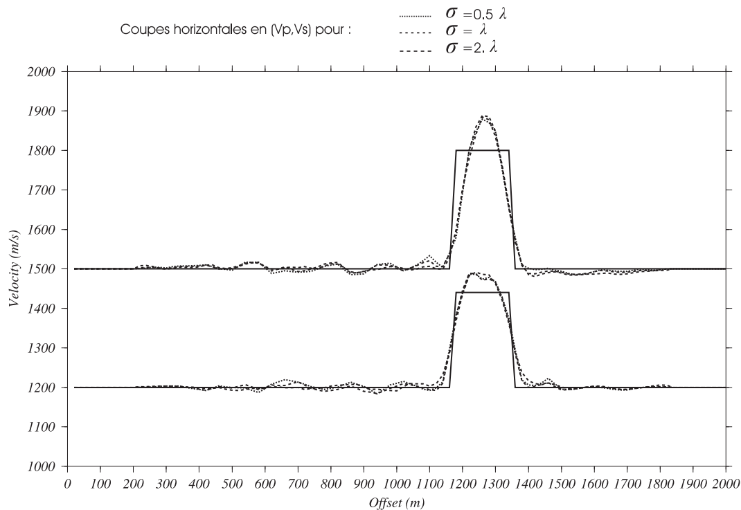
FIG. 4.31: Profils de vitesse horizontaux pour l'inversion de ( V_p, V_s ) avec l'approximation de Born et différentes valeurs de lissage spatial. \sigma est la valeur de la longueur de corrélation de la gaussienne spatiale, \lambda est la longueur d'onde.
