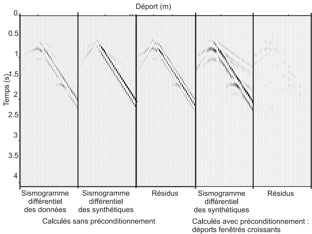
FIG. 4.85: Résidus horizontaux calculés pour une inversion sans (à gauche) et avec preconditionnement par déport croissant (à droite). Les fréquences inversées sont deux fois plus nombreuses que précédemment. Le sismogramme différentiel des données est commun à tous les cas.
