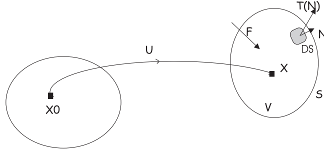
FIG. 2.1: Schéma du déplacement d'un corps dans l'espace et dans le temps. A t=0 , le point matériel \mathbf{x} est en \mathbf{x}_0 . A t>0 , le point matériel est en \mathbf{x} et a effectué un déplacement \mathbf{u} . Le volume V est soumis à des forces volumiques \mathbf{f} et à des forces surfaciques \mathbf{T} s'exerçant sur S , sa surface.
