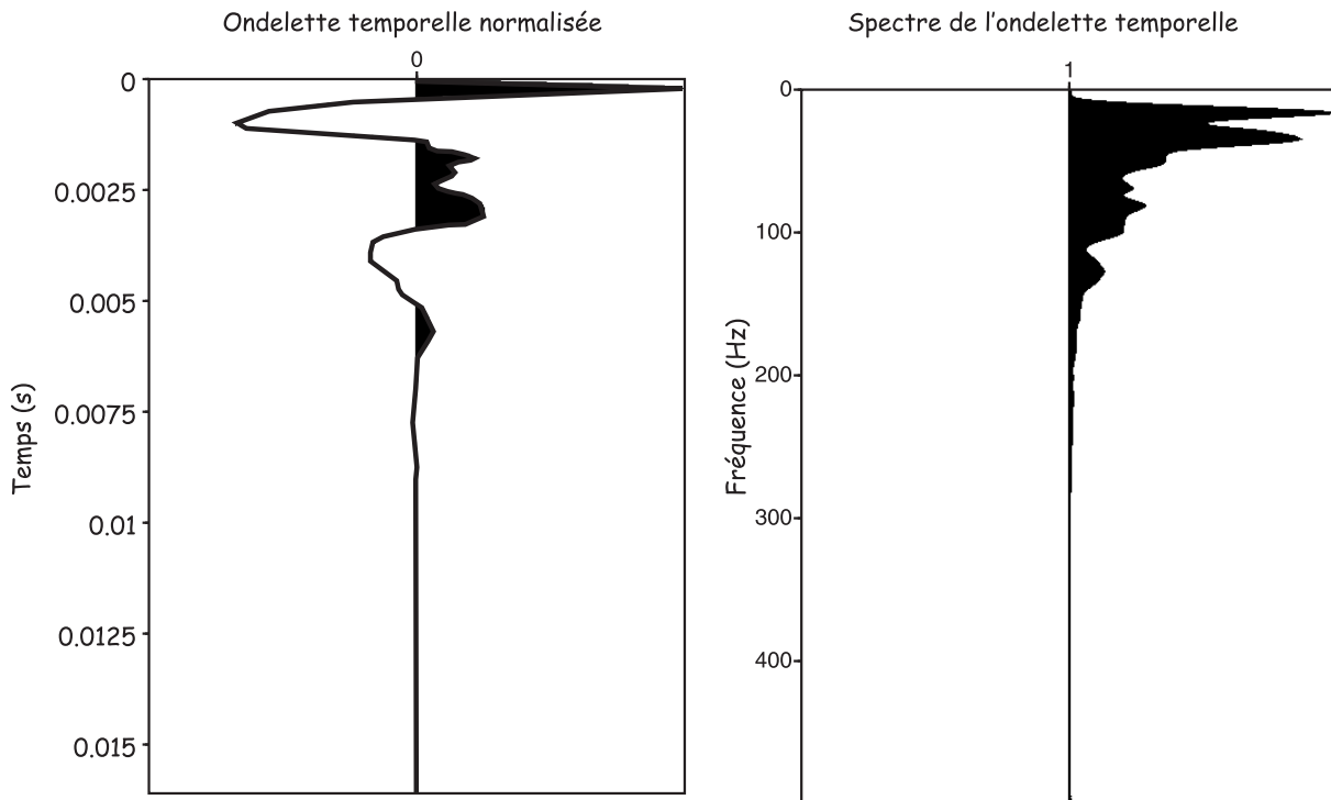
FIG. 5.11: Source temporelle calculée à partir du blanchiment des données et contenu fréquentiel associé
