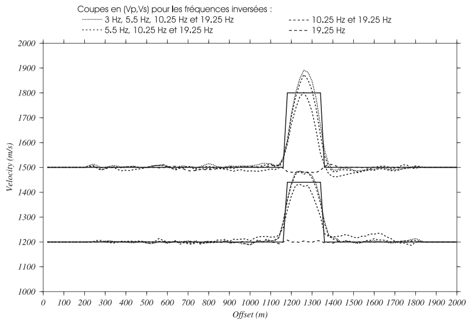
FIG. 4.57: Profils horizontaux extraits des modèles de vitesse pour le cas sans surface libre avec l'approximation de Born, le couple de paramètres inversés ( V_p , V_s ) et un dispositif en transmission. En trait continu : profils extraits des modèles de référence. En trait pointillé : profils extraits des images de l'inversion. La première fréquence inversée augmente et les courbes s'éloignent du modèle vrai.
