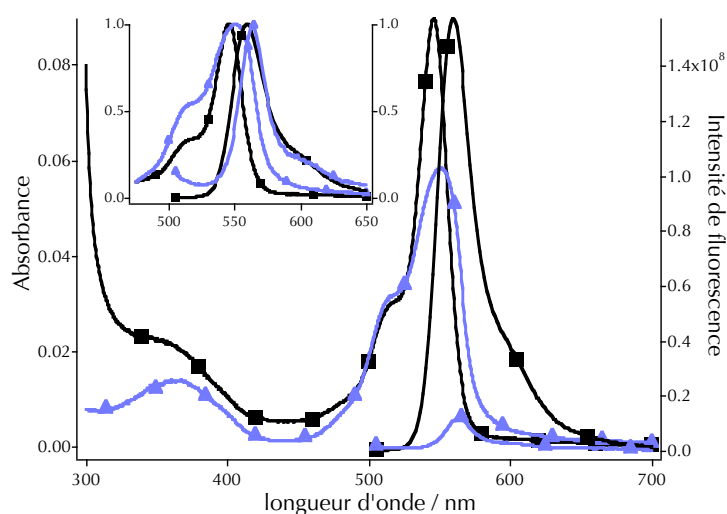
FIG. 9.11 – Spectres d'absorption et de fluorescence des NL-pyr-1 dopés avec du TMB (■) et du blanc correspondant (▲), dilués dans l'eau ( [DTAB] = 0,025\% en masse \ll cmc ). Encart : spectres normalisés.
