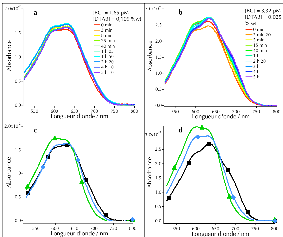
FIG. 9.17 – Spectres d'absorption du BC dilué dans l'eau, en présence de DTAB. a : Évolution du spectre d'absorption d'une solution de BC à 1,65 \mu\text{mol.L}^{-1} en présence de DTAB à 0,109 \text{ \%} en masse ( \approx 0,2 \text{ cmc} ). b : Évolution du spectre d'absorption d'une solution de BC à 3,32 \mu\text{mol.L}^{-1} en présence de DTAB à 0,025 \text{ \%} en masse ( \approx 0,05 \text{ cmc} ). c : BC à \approx 1,63 \mu\text{mol.L}^{-1} , ■ dernier spectre de a ; ▲ : dilution dans l'eau après 24h; ◆ : dilution dans du DTAB à 0,244 \text{ \%} en masse ( \approx 0,5 \text{ cmc} ), après 24h. d : BC à \approx 3,32 \mu\text{mol.L}^{-1} , ■ dernier spectre de b ; ▲ : dilution dans l'eau, après 24h; ◆ : dilution dans le DTAB à 0,244 \text{ \%} en masse, après 24h.
