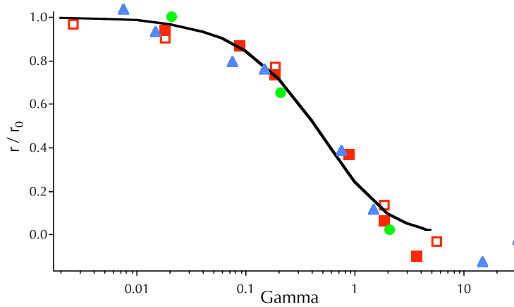
FIG. 8.8 – Évolution du rapport entre l'anisotropie stationnaire et l'anisotropie limite en fonction de \gamma ; — : théorie ; ■ : TMB dans le PMMA à M_w = 120\,000 \text{ g.mol}^{-1} ; □ : TMB dans le PMMA à M_w = 15\,000 \text{ g.mol}^{-1} ; ▲ : PM597 dans le PMMA à M_w = 120\,000 \text{ g.mol}^{-1} ; ● : MB dans le PMMA à M_w = 15\,000 \text{ g.mol}^{-1} .
