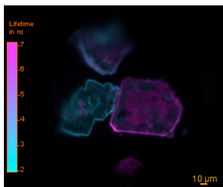
FIG. 4.8 – Image de durée de vie de fluorescence de cristaux de PM597. Les ROI représentées ont servis à reconstruire les déclins de la figure 4.10.
