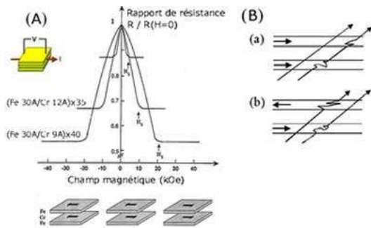
FIG. I.2 – (A) Première observation de GMR avec une magnétorésistance qui s'élève à 80%. (B) Illustration du mécanisme de la GMR. Les lignes obliques représentent des trajectoires d'électrons. Lorsque le spin de l'électron est de même orientation que l'aimantation de la couche, il peut diffuser tandis qu'une orientation contraire le ralentit.
