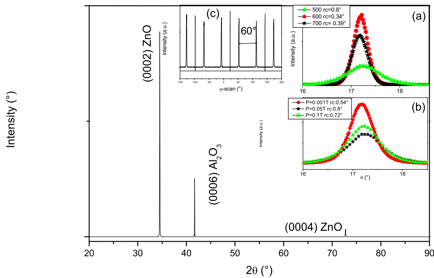
FIG. V.1 – Diagramme de diffraction d'un film Co-ZnO (2% Co) réalisé avec une cible céramique. Le pic de Co-ZnO (0002) étant très intense, il montre une bonne cristallinité du film. En insert, les largeurs à mi-hauteur des réflexions (0002) pour les films avec différentes températures sous PO_2 = 0.05 Torr (a) et différentes pressions d'oxygènes à 500 °C (b). Enfin la relation d'épitaxie est aussi montrée (c).
