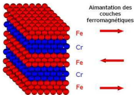
FIG. I.1 – Cette multicouche est semblable à celle de la découverte de la magnétorésistance géante en 1988. Les flèches indiquent l'orientation de l'aimantation des couches de fer avant application d'un champ magnétique.
