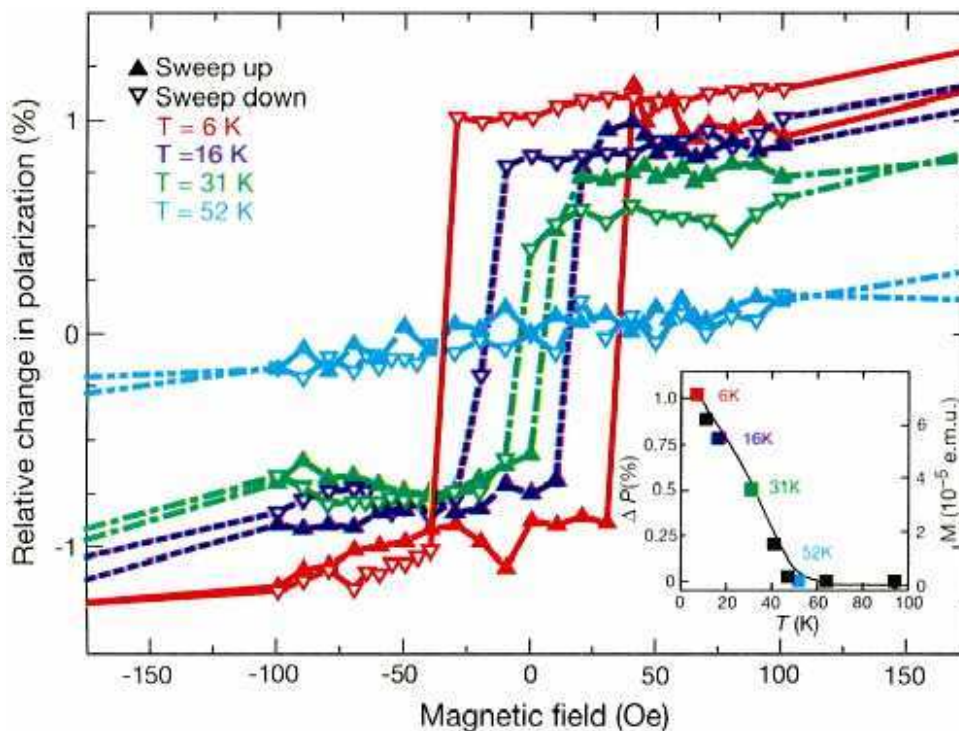
FIG. I.6 – Polarisation électroluminescente de l'injection en spin à partir de GaAs :Mn en fonction du champs magnétique pour différentes températures. En insert : la polarisation rémanente relative et le moment magnétique en fonction de la température
