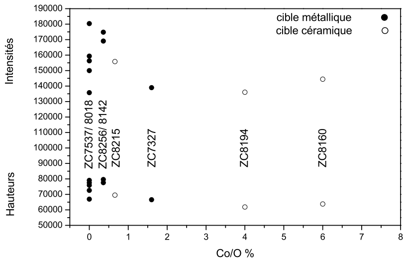
FIG. V.6 Comparaison des intensités et des hauteurs normalisées relatives au niveau 2p^{\frac{3}{2}} du zinc dans les films Zn_{(1-x)}Co_xO
