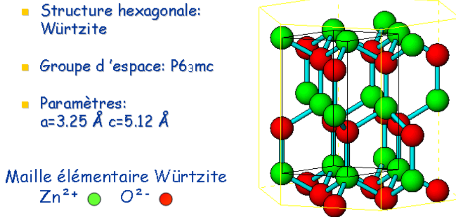
FIG. I.12 – Structure schématique de la wurtzite.
