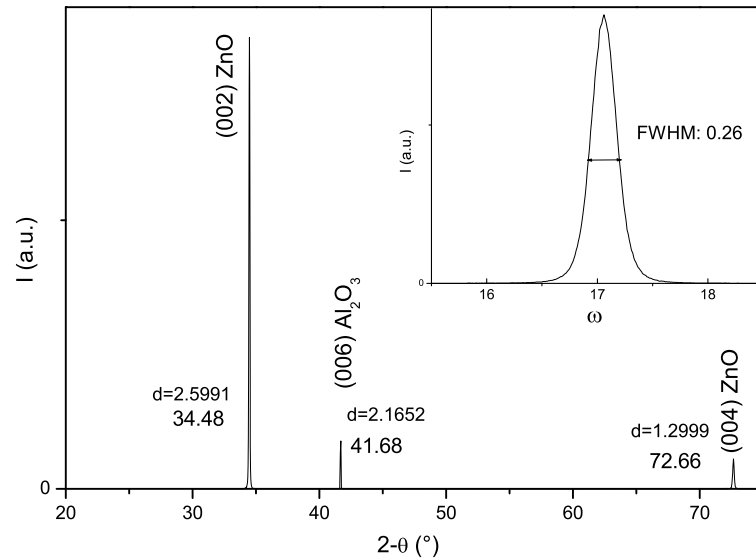
FIG. II.4 – Diagramme de diffraction des rayons X d'un film de ZnO orienté [001] déposé sur un substrat de saphir [001]. En insert : le "rocking curve" de la réflexion (002) du film.
