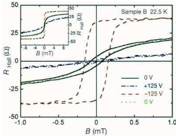
FIG. I.9 – Résistance de Hall ( R_{Hall} ) en fonction du champ magnétique sous trois différentes tensions de grille à 22.5K. En insert : les mêmes courbes montrées à des champs magnétiques plus importants.
