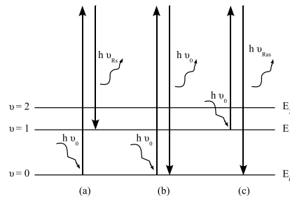
FIG. 1.10 – (a) Diffusion Raman Stokes ( \nu_{R_s} = \nu_0 - \nu_a ), (b) Diffusion élastique, (c) Diffusion Raman anti-Stokes ( \nu_{R_{as}} = \nu_0 + \nu_a ), avec \nu_0 la fréquence de la source monochromatique excitatrice du spectre. Si le photon incident a une énergie très supérieure au niveau d'énergie de vibration, alors on observe un phénomène de diffusion :
