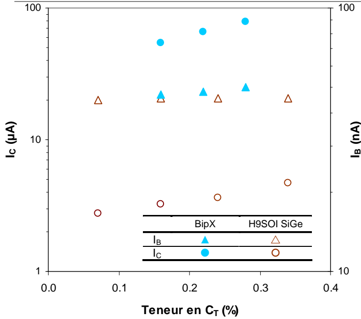
Figure V-8 : Courant collecteur et de base en fonction de la composition en carbone des bases SiGeC:B, dans le cas d'une technologie BipX ( [B]=5.10^{19}at./cm^3 ) et H9SOI SiGe ( [B]=7.10^{19}at./cm^3 ). Le système utilisé est SiH 4 /GeH 4 /MS/HCl/B 2 H 6 /H 2 .
