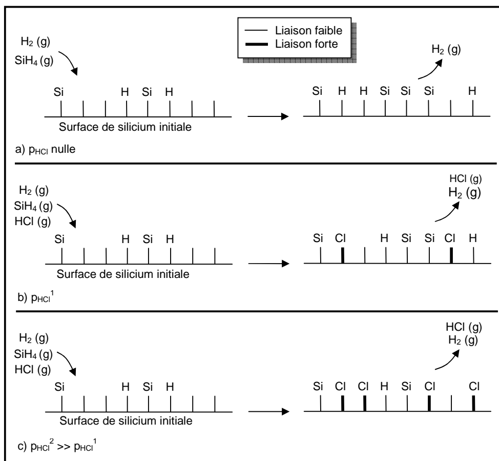
Figure II-6 : Schéma de réactions susceptibles d'être présentes à la surface de croissance silicium pour un système \text{SiH}_4/\text{HCl}/\text{H}_2 .
