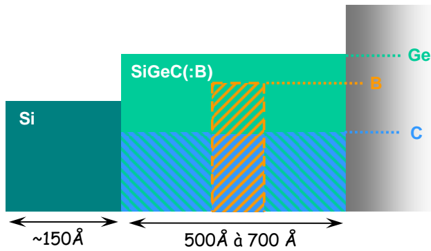
Figure IV-2 : Profil standard des films \text{Si}/\text{SiGeC}:\text{B} élaborés pour déterminer les concentrations en carbone total et substitutionnel et pour simuler la diffusion du dopant.
