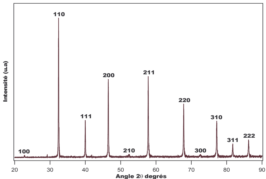
Fig. 2 : Diagramme de diffraction des rayons X par la poudre de SrTiO 3 .
