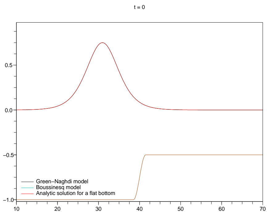
FIG. 7.2.9 – Résultats obtenus pour \mu = 0.05 , \varepsilon = 0.2 et \beta = 0.5
