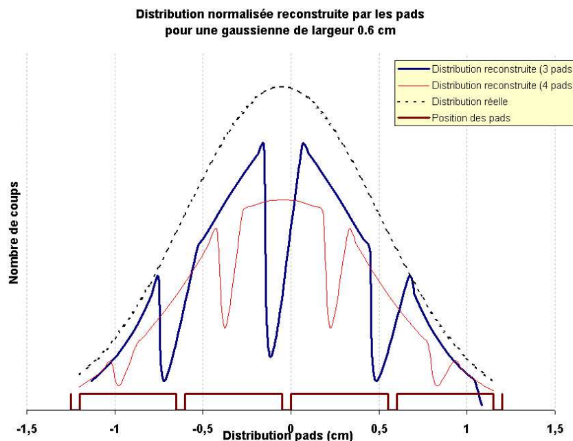
FIG. 3.3 – Reconstruction simulée d'une distribution gaussienne par la méthode de barycentre simple effectuée sur 3 ou 4 pads. Des facteurs multiplicatifs sur l'amplitude des distributions ont été appliqués pour des raisons de lisibilité.
