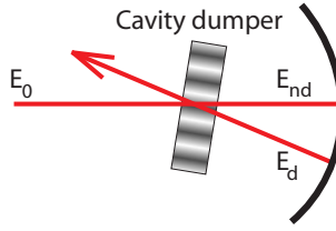
Figure 3.6: Extraction d'impulsions par cavity dumper à double passage.
