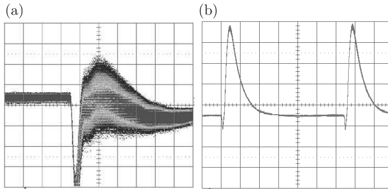
Figure 3.18: Réponse homodyne typique : (a) Lorsque les voies sont équilibrées (échelle H : 50 \text{ ns/div} , V : 50 \text{ mV/div} ); (b) Lorsque les voies sont déséquilibrées ( H : 200 \text{ ns/div} , V : 500 \text{ mV/div} ).
