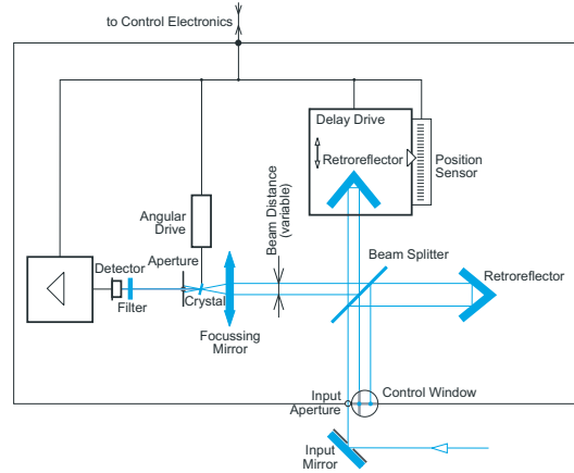
Figure 3.9: Principe de fonctionnement de l'autocorrélateur APE PulseCheck.
