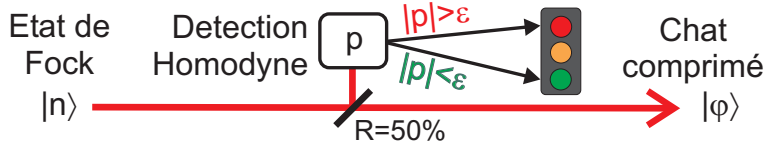
Figure 6.1: Protocole utilisé pour la préparation de “chats comprimés”. Un état de Fock |n\rangle est divisé sur une lame 50/50. Dans le mode réfléchi, on mesure la quadrature \hat{p} . Si le résultat p de la mesure est assez proche de 0, avec un certain seuil de tolérance ( |p| \leq \epsilon \ll 1 ), le mode transmis est préparé dans un état qui reproduit avec une fidélité supérieure à 99% un chat de taille |\alpha|^2 = n , de même parité que n , comprimé de 3 dB suivant x . Dans le cas contraire, on considère que la préparation a échoué, et on recommence la procédure.
