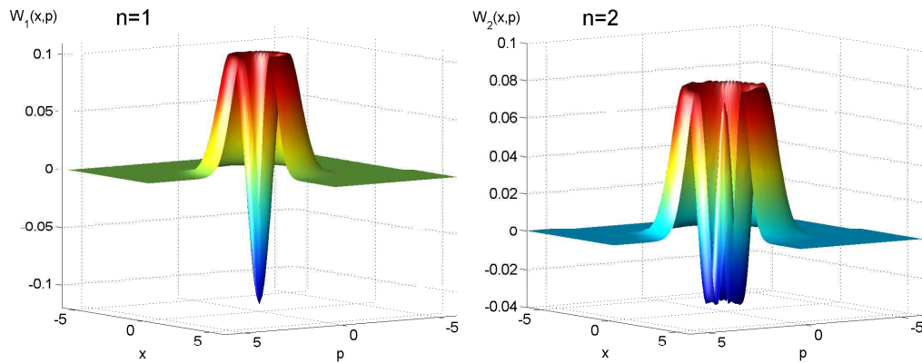
Figure 4.8: Fonctions de Wigner d'états à un et deux photons générés expérimentalement, reconstruites par maximum de vraisemblance, corrigées des pertes homodynes.
