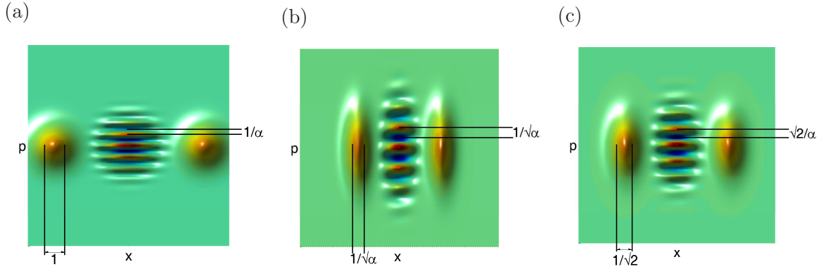
Figure 6.7: (a) Fonction de Wigner d’un chat non comprimé de taille |\alpha|^2 = 10 : la plus petite échelle de variation vaut 1/\alpha , ce qui fixe un maximum pour les fluctuations de bruit qu’il peut subir. (b) Fonction de Wigner du même chat comprimé de s = 1/\alpha : la plus petite échelle de variation vaut maintenant 1/\sqrt{\alpha} , on gagne ainsi un facteur \sqrt{\alpha} en robustesse. (c) Le même état comprimé de 3 dB : lorsque |\alpha|^2 \geq 2 , cette compression augmente la résistance au bruit.
