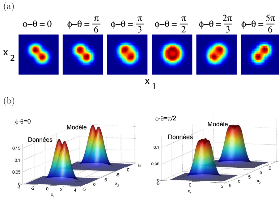
Figure 8.11: (a) Distributions de quadratures jointes P_{\theta,\phi}(x_1, x_2) de l'état de Bell mesurées expérimentalement, tracées pour -3,5 \leq x_1, x_2 \leq 3,5 . (b) Comparaison entre les distributions obtenues directement à partir des données, et celles reconstruites à l'aide du modèle analytique.
