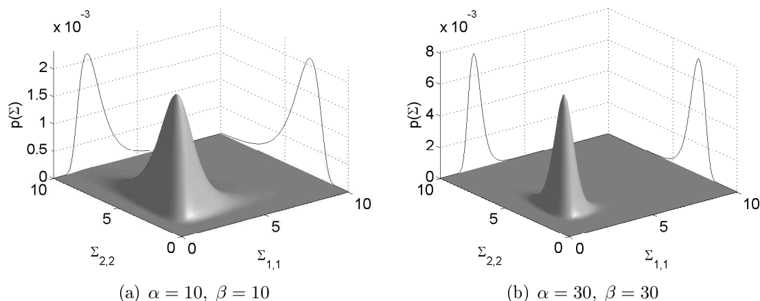
FIG. 3.8 – Loi de Wishart inverse p(\Sigma) d’une matrice diagonale \Sigma . Les traits continus correspondent aux projections de la loi de Wishart inverse dans les plans (\Sigma_{1,1}, 0) et (0, \Sigma_{2,2}) . La densité de probabilité est donnée par p(\Sigma) = p(\Sigma|\alpha, \beta, J) \propto \det(\Sigma^{-1})^\beta \exp[-\alpha \text{Tr}(\Sigma^{-1} J)] , avec dans notre exemple J = \text{diag}(2, 3) (cf. Annexe A).
