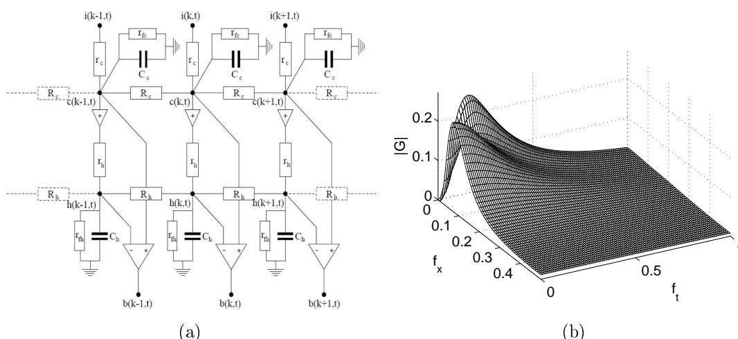
FIG. 4.5 – Rétine artificielle. Figure 4.5(a) : schéma électrique équivalent de la rétine d'après [67, 11]. Figure 4.5(b) : réponse en fréquence spatio-temporelle de G(z_s, f_t) (4.29) où \alpha_c = 2 , \beta_c = 0 , \tau_c = 1 , \alpha_h = 10 , \beta_h = 0 , \tau_h = 1 .
