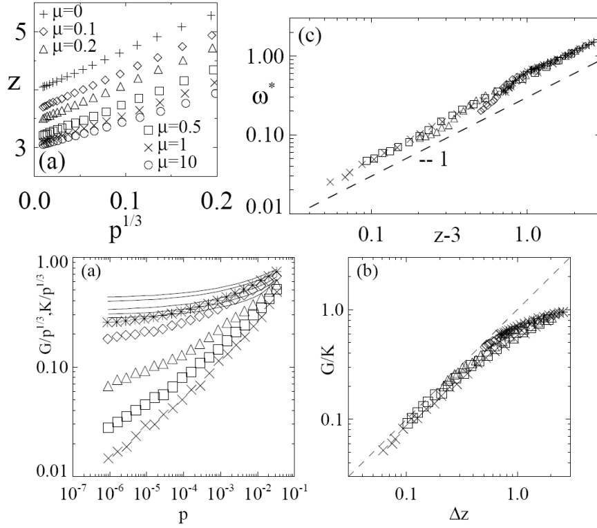
FIG. 1.4: En haut à gauche, coordination moyenne z en fonction de la pression pour différentes valeurs du coefficient de frottement \mu . En haut à droite, fréquence caractéristique des modes anormaux \omega^* en fonction de l'écart à l'isostaticité \Delta z pour différentes valeurs de \mu . En bas, dépendance des modules élastiques de cisaillement G et de compression K à la pression et à \Delta z [48].
