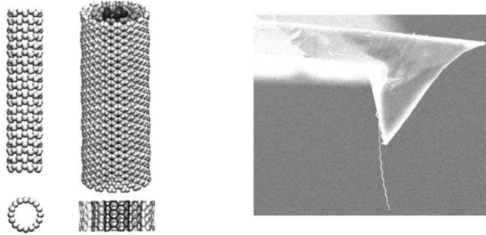
FIG. B.1: A gauche, nanotubes monoparoï et multiparoï (figure adaptée de la référence [306]) A droite, nanotube de carbone multiparoï fixé sur une pointe de microscopie à force atomique [307].
