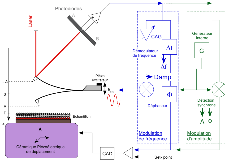
FIG. 1.1: Diagramme schématisé d'un microscope à force atomique dynamique opérant en modulation d'amplitude ou en modulation de fréquence. Le contrôle automatique de déplacement (CAD) permet d'asservir la position de l'échantillon pour maintenir un signal constant, l'amplitude A ou la phase \phi pour la modulation d'amplitude, le déplacement de fréquence \Delta f ou la dissipation Damp pour la modulation de fréquence.
