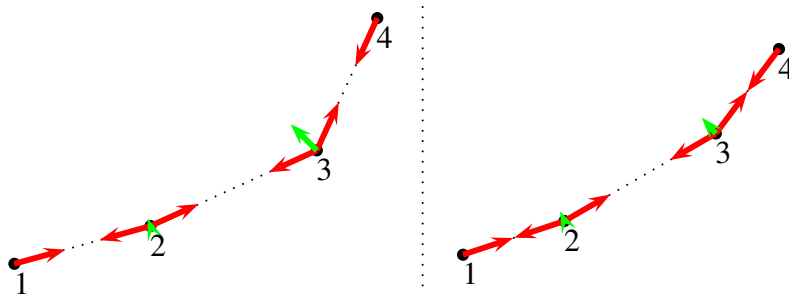
FIGURE 4.35 – Illustration du mécanisme des forces réparties sur une macro-fibre composée de 4 nœuds. À gauche, en début de contraction, à droite en cours de contraction. Sur les nœuds extérieurs 1 et 4 représentant les extrémités de la fibre, une force d'intensité F est appliquée dans la direction de la fibre, vers l'intérieur du muscle. Sur les nœuds intérieurs 2 et 3 sont représentés les deux vecteurs forces agissant sur chaque nœud et leurs résultantes. La norme de la résultante diminue avec l'alignement des nœuds, jusqu'à devenir nulle lorsque les nœuds sont parfaitement alignés.
