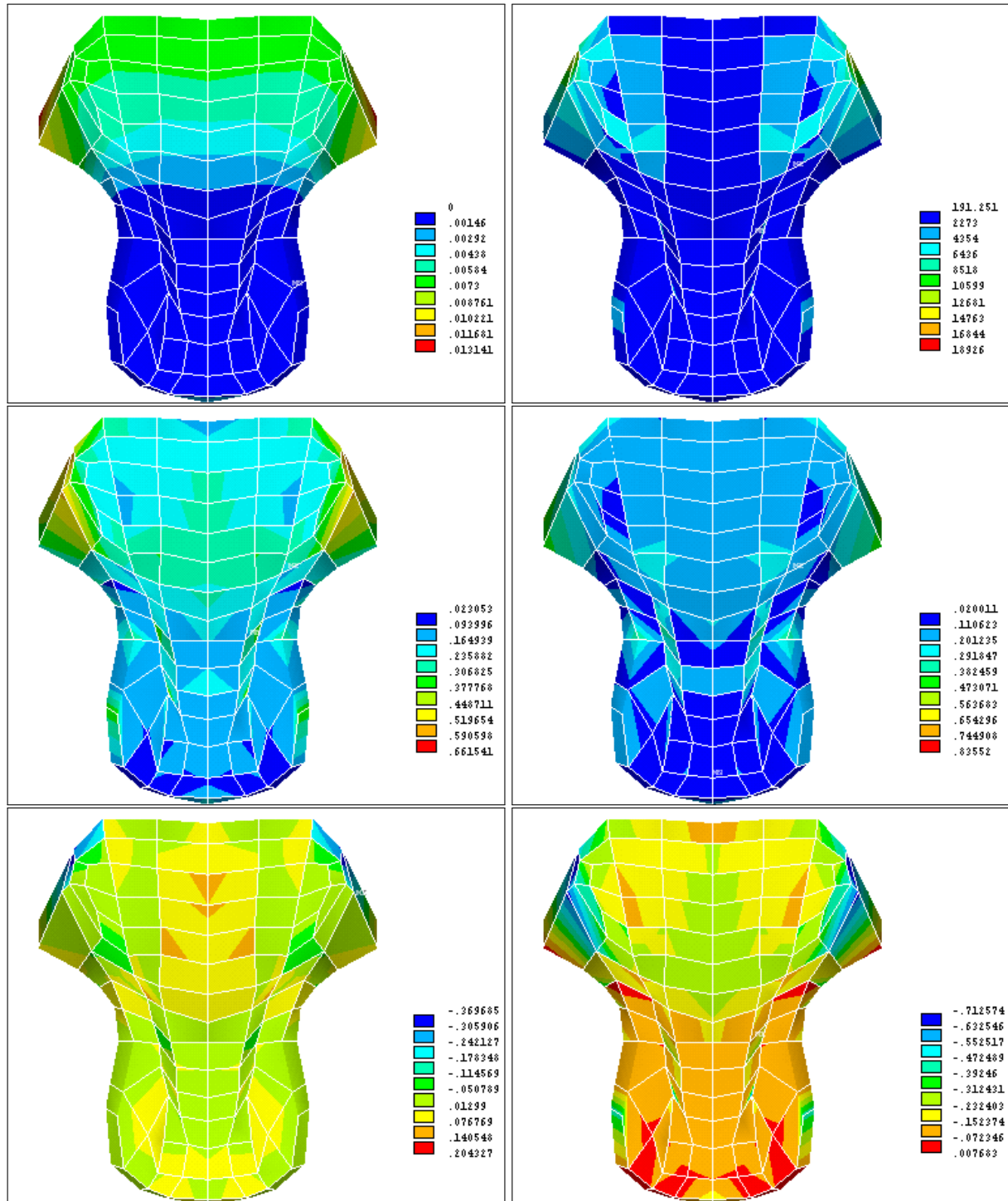
FIGURE B.29 – Cartes des déplacements, des contraintes et des déformations pour la voyelle /a/ dans un plan “coronal”. En haut : à gauche, carte des déplacements (mètres), à droite, carte des contraintes de von Mises (Pa). Au milieu : à gauche, carte des déformations de von Mises (adimensionnelles), à droite, carte des premières déformations principales. En bas : à gauche, carte des secondes déformations principales, à droite, carte des troisièmes déformations principales.
