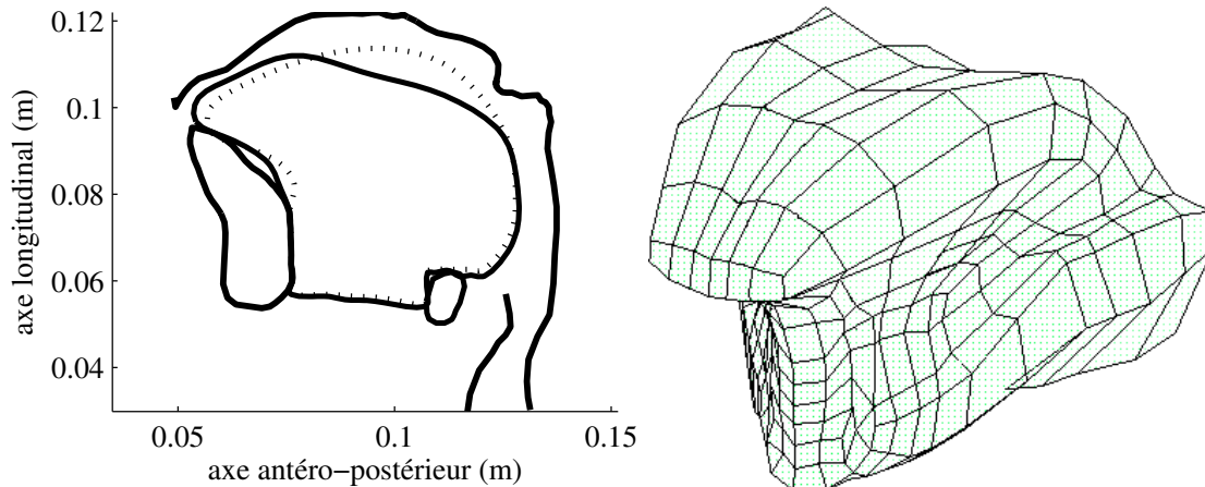
FIGURE 6.3 – Action du génio-glosse médium ( \lambda_{GGm} = 0,75 \times l_{GGm} ). Contour des articulateurs linguau dans le plan médiosagittal (gauche, les pointillés représentent la position de repos) et vue oblique de la langue (droite).
