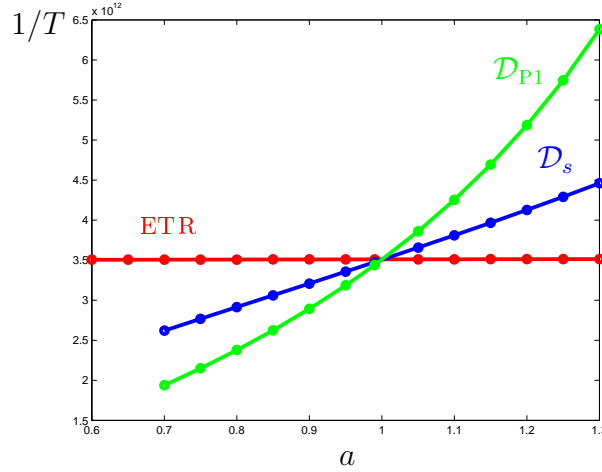
FIG. III.4 – Comparaison des pentes des logarithmes des flux transmis aux temps longs en fonction de l'albédo a pour un facteur d'anisotropie g = 0.5 (fonction de phase d'HENYEY-GREENSTEIN), une longueur de diffusion l_s = 4.75 \times 10^{-7} m, des indices optiques tous égaux n_1 = n_2 = n_3 = 1 et une épaisseur de milieu de L = 1.5 \times 10^{-5} m pour le calcul ETR et l'approximation de la diffusion ( \mathcal{D}_s asymptotique en régime stationnaire et \mathcal{D}_{P1} en approximation P1).
