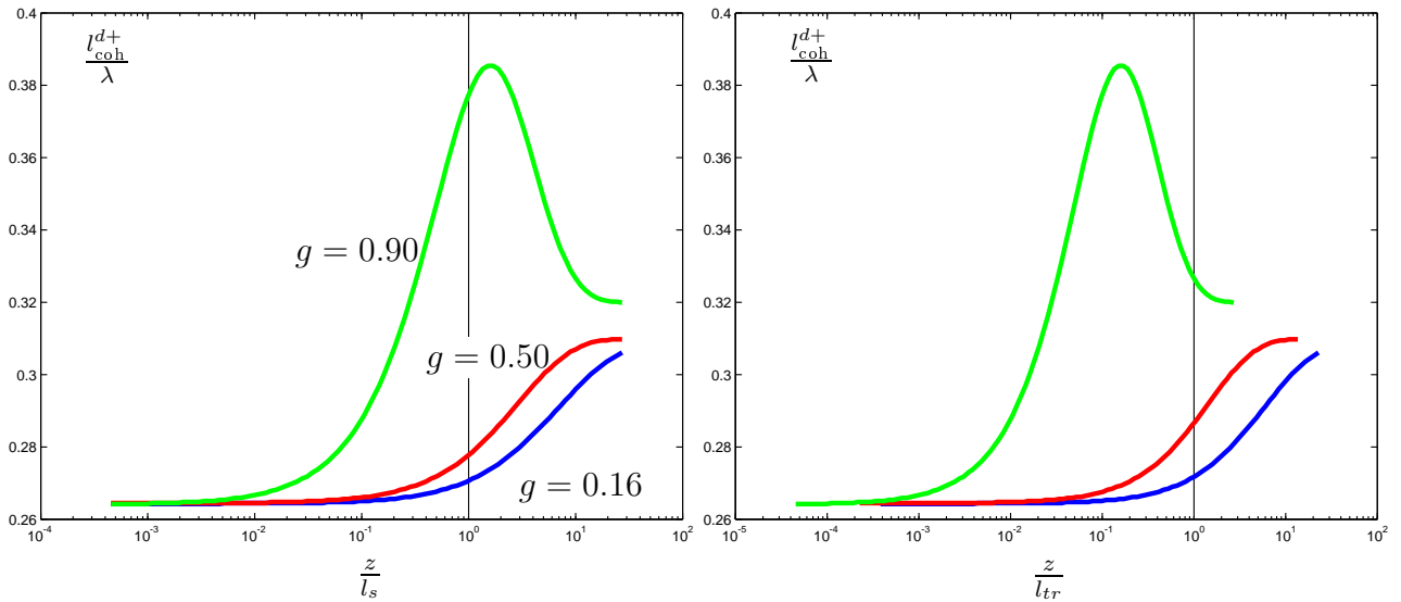
FIG. II.8 – Tracé de la longueur de cohérence l_{coh}^{d+} correspondant à la luminance diffuse vers l'avant avec n_2 = 1.33 en fonction de la profondeur z dans le milieu normalisée par la longueur de diffusion (figure de gauche) et par la longueur de transport (figure de droite).
