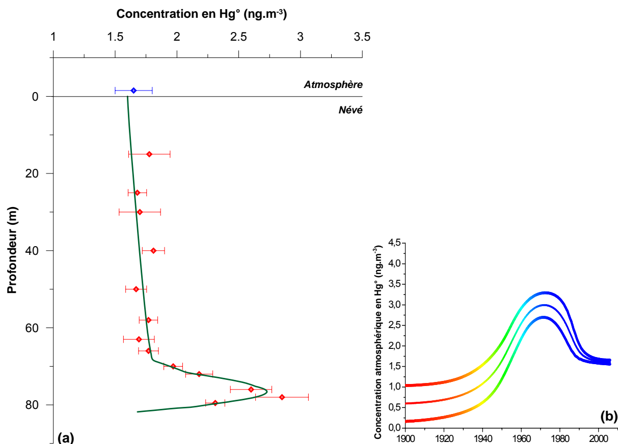
Figure IV.20. Diffusion dans le névé du scénario moyen reconstruit pour \text{Hg}^\circ (a). Le scénario moyen est représenté en (b) au centre de l'enveloppe.
