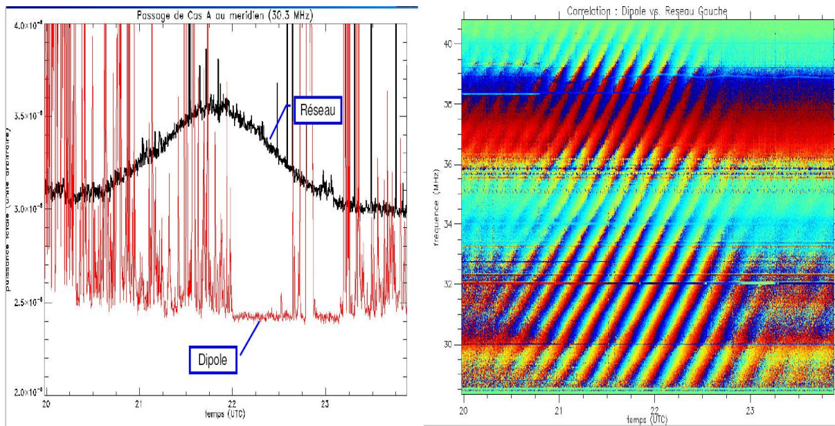
FIG. A.10 – Figures extraite de [84]. A gauche le transit d'une source radio (Cyg-A) en fonction du temps observé avec le réseau du DAM de Nançay (en noir), le dipôle court (en rouge) ne voit pas d'excès significatif. A droite, les franges d'interférences des 2 instruments (DAM et dipôle) en fonction du temps indiquant que le dipôle est sensible au passage de la radio source car les franges d'interférences couvrent la totalité de l'intervalle de temps de transit de la radio source dans le ciel.
