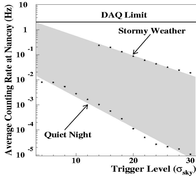
FIG. 6.6 – Taux de déclenchement de l'expérience CODALEMA à Nançay en fonction du seuil exprimé en nombre de \sigma_{sky} , l'écart type du bruit mesuré dans la bande de fréquence du trigger. Le taux de déclenchement, zone grisée, varie en fonction des conditions extérieures. Les valeurs atteintes ( < 1 Hz) sont prometteuses pour envisager un fonctionnement autodéclenché de la radiodétection des gerbes atmosphériques.
