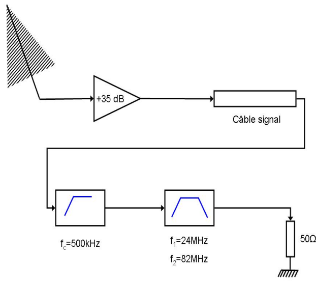
FIG. 4.7 – Chaîne d'acquisition pour une antenne sur CODALEMA. Le signal d'antenne est tout d'abord amplifié de 35 dB avant d'être transmis par les câbles jusqu'au centre d'acquisition. Deux filtrages successifs sont ensuite appliqués aux signaux, le premier est un passe-bas de 500 kHz destiné à atténuer l'émetteur France Inter grandes ondes, le second un passe-bande de 24-82 MHz qui permet de compenser la résolution de l'ADC. Les signaux sont finalement numérisés sur un oscilloscope numérique.
