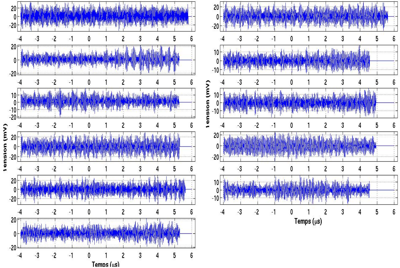
Figure 4.12: Évènement typique enregistré sur CODALEMA. Les signaux d’antennes sont enregistrés en fonction du temps sur 10 \mu\text{s} dans la bande de fréquence 24\text{--}82 \text{ MHz} . Le zéro du temps est donné par l’instant de déclenchement de l’acquisition. De haut en bas et de gauche à droite les antennes : L0 , L1 , L2 , NE , SE , NW , SW , L5 , L3 , L4 , L6 .
