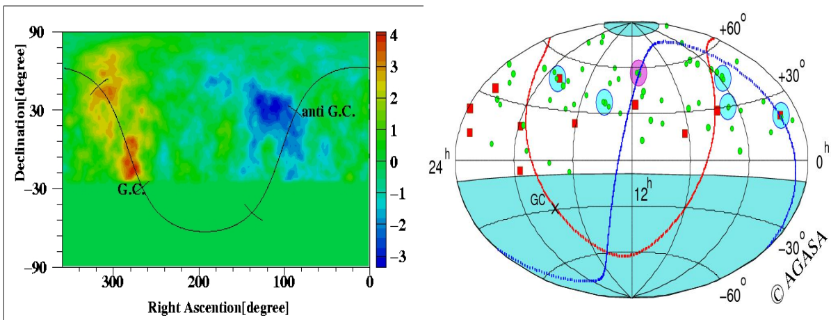
FIG. 2.7 – A gauche, figure extraite de [34] présentant l’anisotropie mesurée sur AGASA à 10^{18} \text{ eV} . On observe un excès significatif d’évènements en direction du centre galactique et un déficit vers l’anti-centre. A droite, figure extraite de [35], la distribution des évènements détectés sur AGASA au dessus de 4 \cdot 10^{19} \text{ eV} présente des doublets et un triplet dont la probabilité d’occurrence est estimée à moins de 1%.
