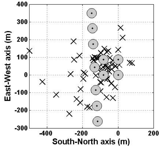
FIG. 5.32 – Localisation des coeurs de gerbes pour les 58 événements reconstruits sur le réseau d'antennes CODALEMA. Les antennes sont symbolisées par des cercles grisés et les positions des coeurs par des croix.
