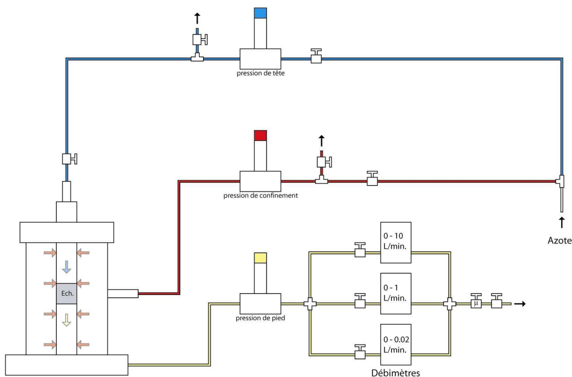
Figure II.5 : Dispositif de mesure de la perméabilité.
