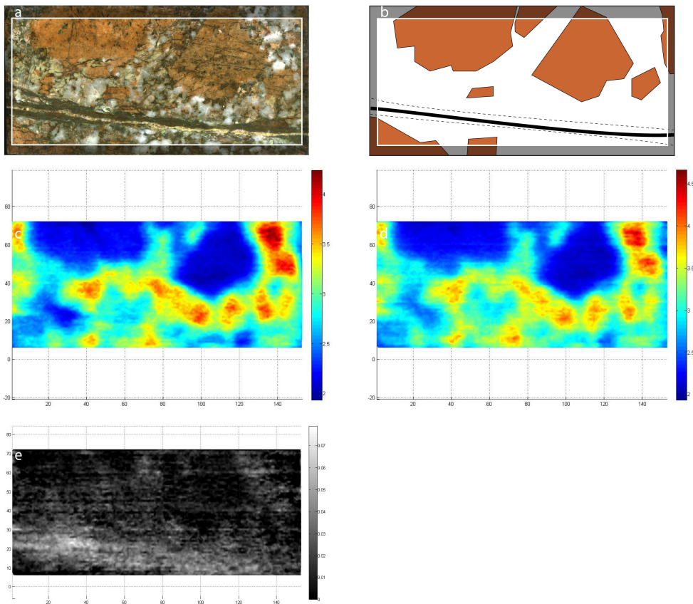
(a) photo de l'échantillon et délimitation de la zone scannée, (b) schéma minéralogique et structural, (c) carte de conductivité thermique de l'échantillon sec, (d) carte de conductivité thermique de l'échantillon saturé, (e) carte de densité de porosité.
