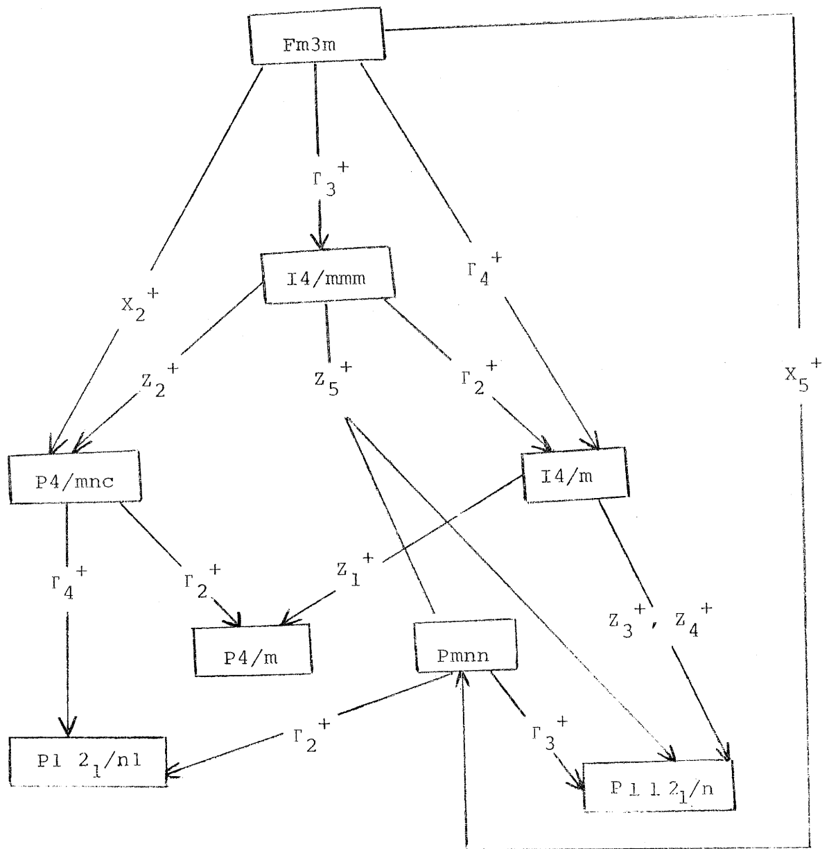
Fig. 36 - Relations de groupes à sous-groupes et transitions de phase possibles de Rb_2KFeF_6 et Rb_2KYF_6 .
