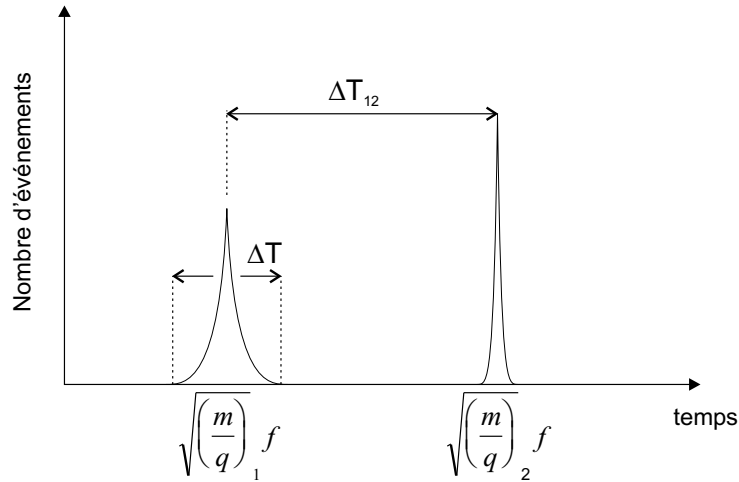
FIG. 3.4 – Le spectre de temps de vol mesuré des ions se présente sous la forme d'un ensemble de pics correspondant chacun à des particules ayant un même rapport m/q .
