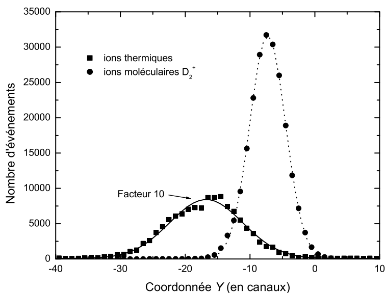
FIG. 4.15 – Distribution des positions d'impact des ions thermiques et des ions D_2^+ , suivant la direction du jet. Le décalage mesuré entre ces deux distributions permet de déterminer la vitesse d'entraînement des molécules dans le jet.
