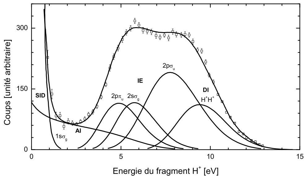
FIG. 1.4 – Distribution d'énergie des fragments H^+ produits par les différents processus d'ionisation dissociative (SID, AI, IE et DI) mesurée par Edwards et al. [EWDE90, EWDE91]. Les données expérimentales sont ajustées par les distributions d'énergie obtenues par la méthode des projections [CJP36], pour quelques états de H_2^{**} , de H_2^+ ( 1s\sigma_g , 2p\pi_u , 2s\sigma_g , 2p\sigma_u ) et de H_2^{2+} ( H^+H^+ ).
