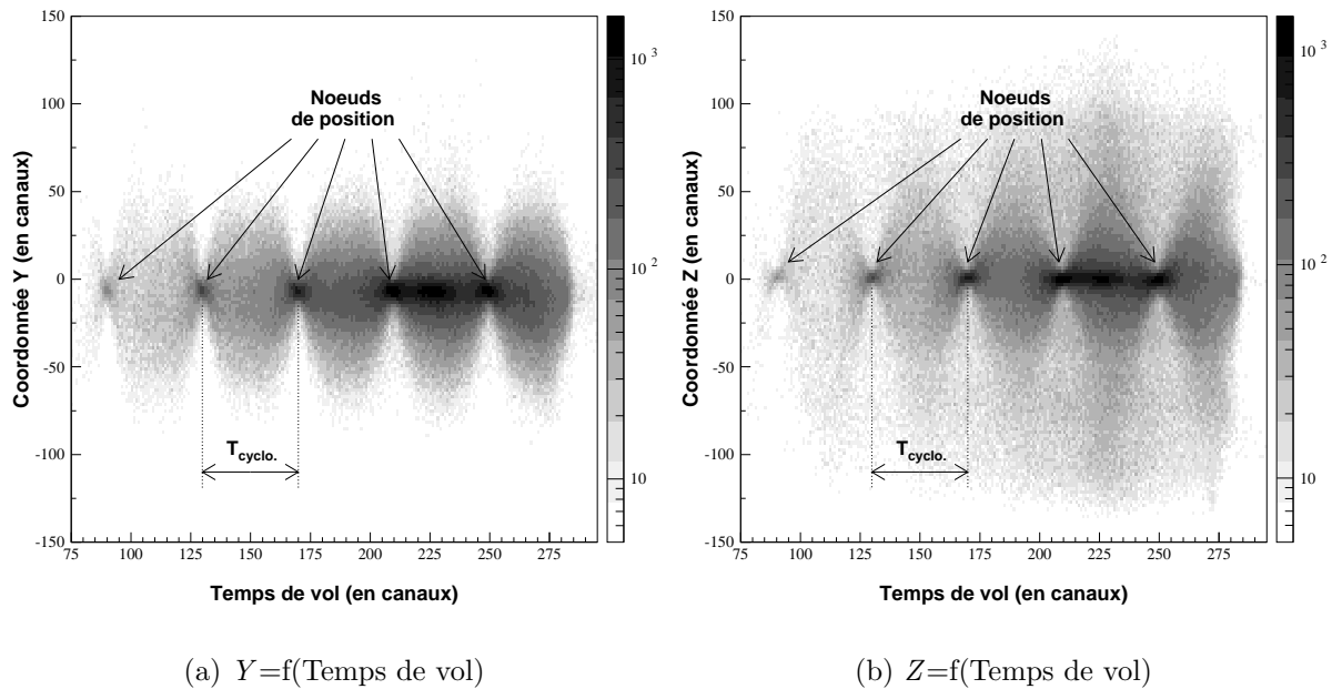
FIG. 4.12 – Détermination de l'origine des positions. Les noeuds de positions observés pour les temps de vol égaux à un nombre entier de période cyclotronique ( T_{cyclo.} ) correspondent à la position initiale d'émission des électrons (origine des positions).
