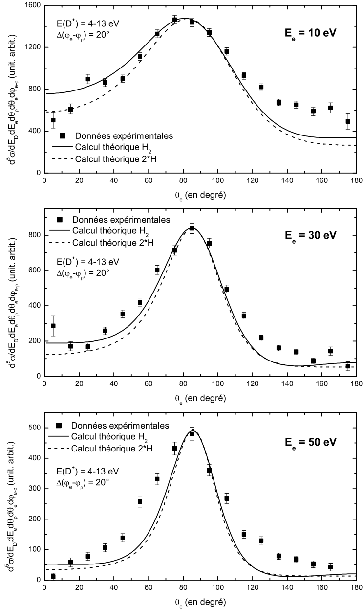
FIG. 5.17 – Distributions angulaires des électrons d'énergie égale à 10, 30 et 50 eV, pour une orientation de l'axe moléculaire perpendiculaire à la direction du projectile ( \theta_\rho = 90 degrés). Les données expérimentales (représentées par les points) sont comparées aux résultats théoriques obtenus par la méthode CDW-EIS (les courbes continue et discontinue représentent respectivement les cas moléculaire et atomique).
