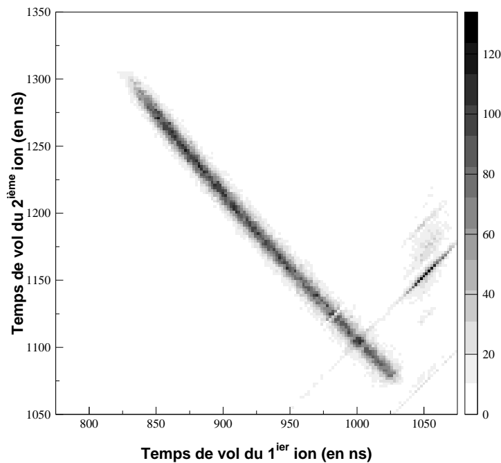
FIG. 4.17 – Temps de vol de l'ion D^+ émis à l'opposé du détecteur ( 2^{\text{ième}} ion détecté), en fonction du temps de vol de l'ion émis vers le détecteur ( 1^{\text{er}} ion détecté). La corrélation observée découle directement de la conservation de la quantité de mouvement gouvernant la dissociation de l'ion moléculaire D_2^{2+} .
